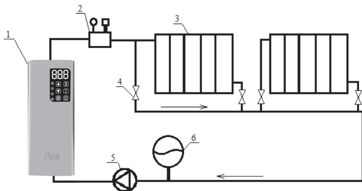
Рисунок 7.1. Примерная схема однотрубной системы отопления с принудительной циркуляцией.
