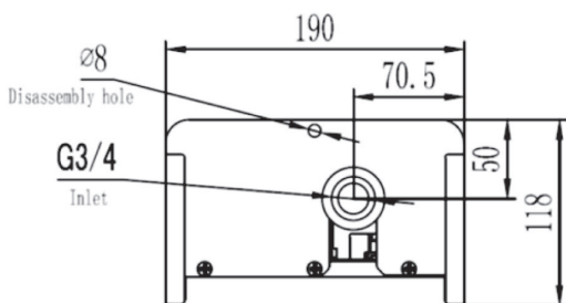
Рисунок 4.1. Габаритные размеры для подключения к системе отопления ES-3, ES-5.
