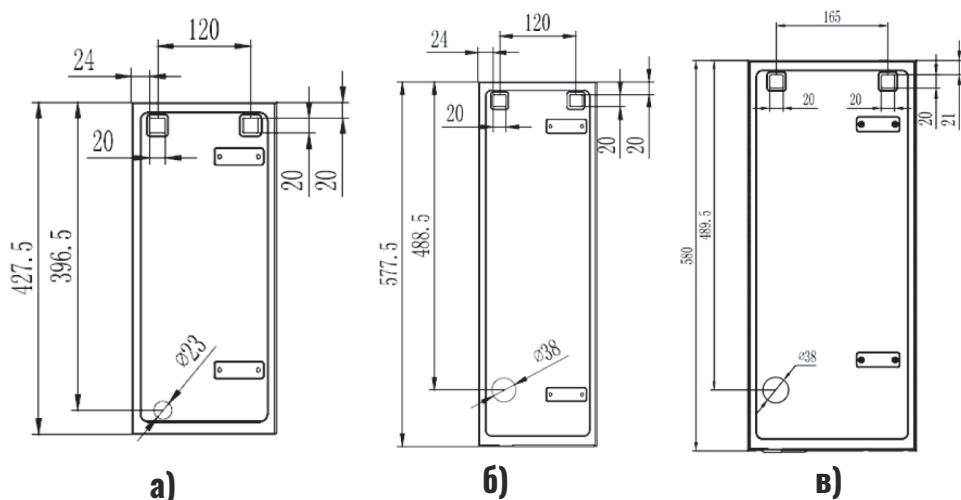
Рисунок 3. Монтажные размеры для крепления на стены.
