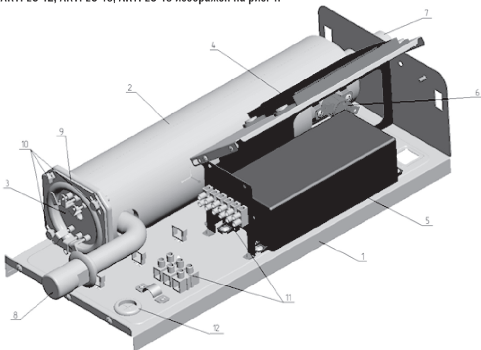
Рисунок 1. Котел отопительный электрический ES-3, ES-5, ES-6, ES-8, ES-9, ES-12, ES-15, ES-18
