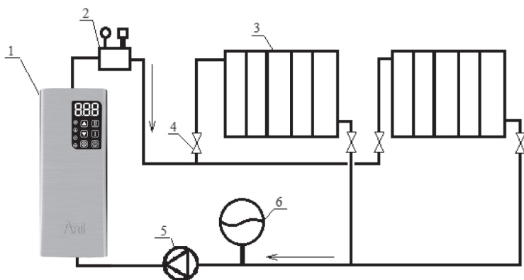
Рисунок 7.2. Примерная схема двухтрубной системы отопления с принудительной циркуляцией.
