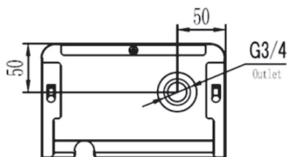
Рисунок 4.2. Габаритные размеры для подключения к системе отопления ES-6, ES-8, ES-9, ES-12, ES-15, ES-18.
