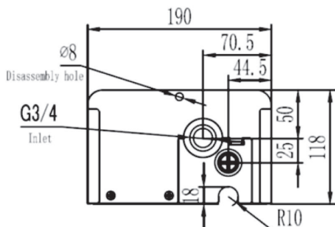
Рисунок 4.2. Габаритные размеры для подключения к системе отопления ES-6, ES-8, ES-9, ES-12, ES-15, ES-18.
