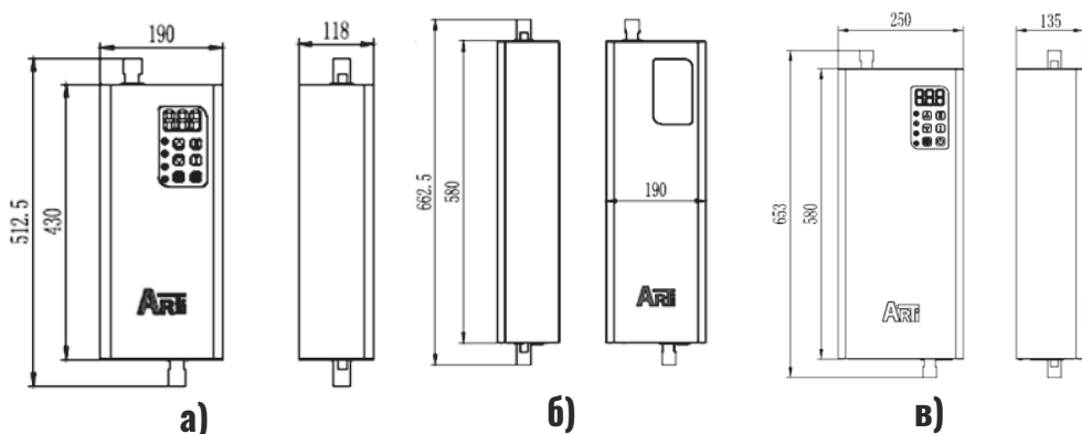
Рисунок 2. Габаритные размеры.
