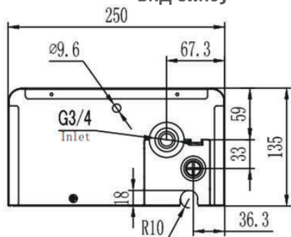
Рисунок 4.3. Габаритные размеры для подключения к системе отопления ES-15, ES-18.
