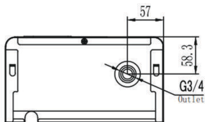
Рисунок 4.3. Габаритные размеры для подключения к системе отопления ES-15, ES-18.
