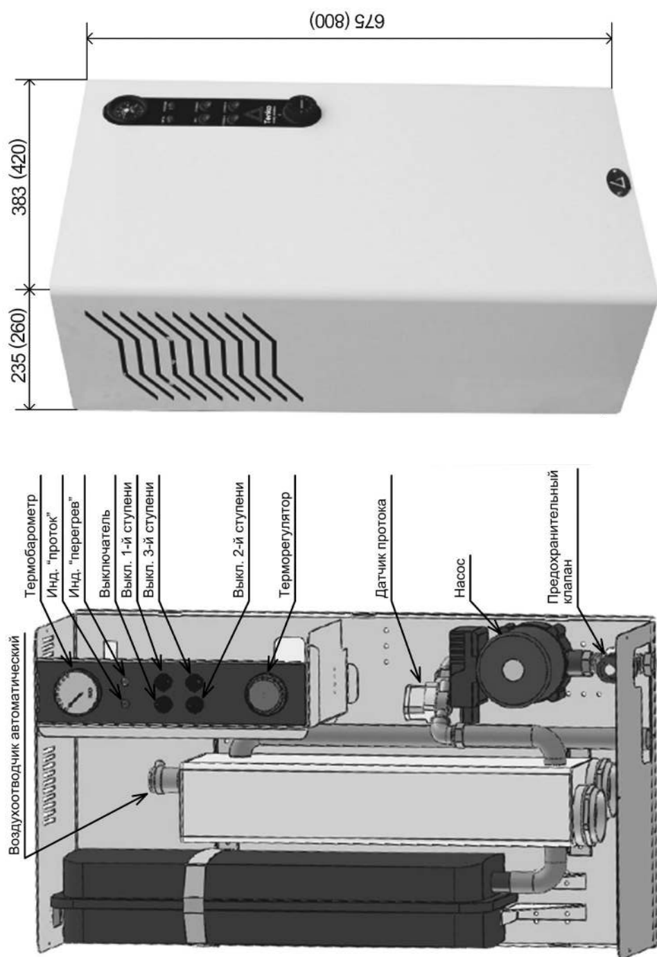
Рис. 3. Внешний вид электродотла Тенко «Стандарт ПЛЮС»
