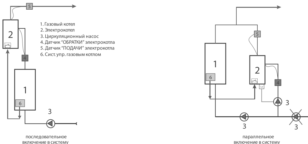
Рис. 11. Комбинированное отопление. Схемы подключения электрокотла.
