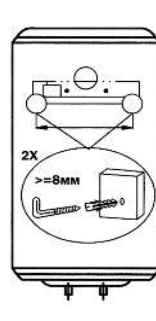
в) модель E-series (N4E, N4L), O'Pro (N4), EGO (D400-1-M), O'ProP, O'Pro+ (D 400-1 M), Steatite S4 CM - вертикальні, Steatite D400-2-BC, D325-2-BC), EXPERT, TURBO
