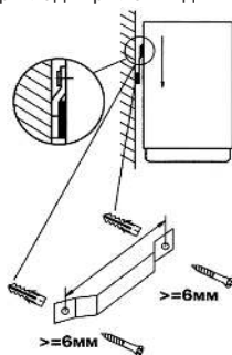
а) модель O'pro (PC, S3S), Steatite (S3C)
