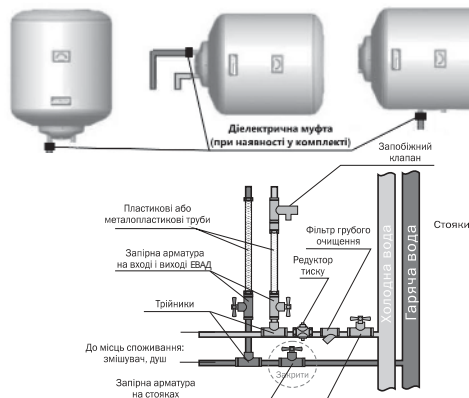
Рис. 5. Підключення ЕВАД у вертикальному / горизонтальному положенні
