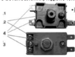
в) модель O'Pro (S3S), EXPERT, TURBO, Steatite (S3C, S4CM, D400-2-BC, D325-2-BC)
