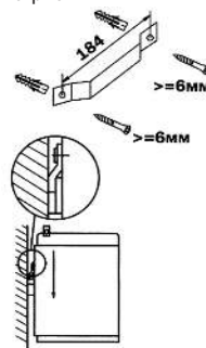
б) модель O'Pro (PC 10SB/15S)
