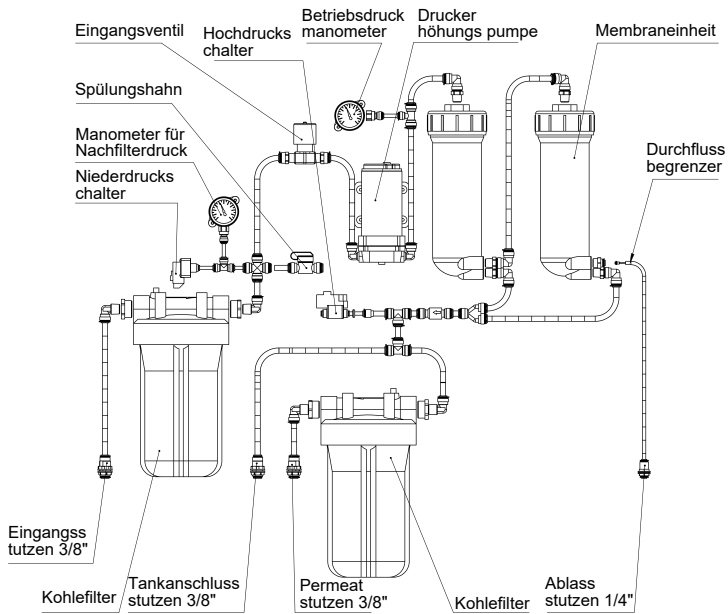
Abbildung 5. Schema des Systems ROust 3000
