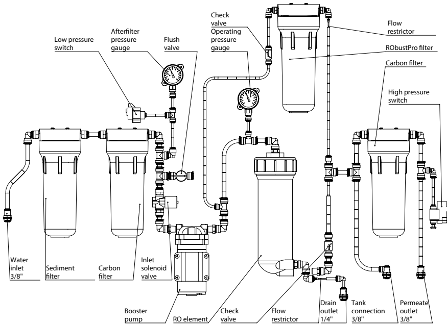
Abbildung 4. Schema des Systems ROust PRO
