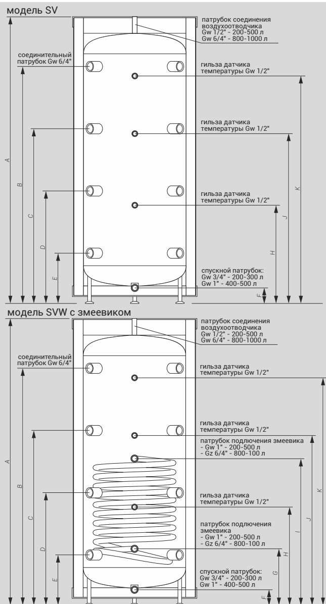
SV/SVW 200-500 л
