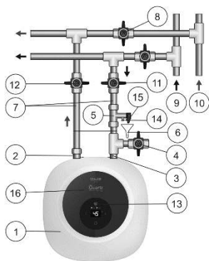
Малюнок 1. Схема підключення ЕВН до водопроводу для моделей Vallon U (патрубки вверху) та Vallon O (патрубки униз)
