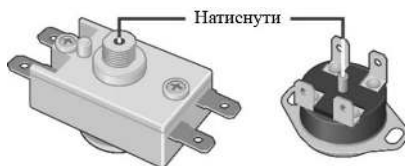
Малюнок 2. Схема розташування кнопки термовимикача. Зовнішній вигляд термовимикача залежить від моделі обладнання
