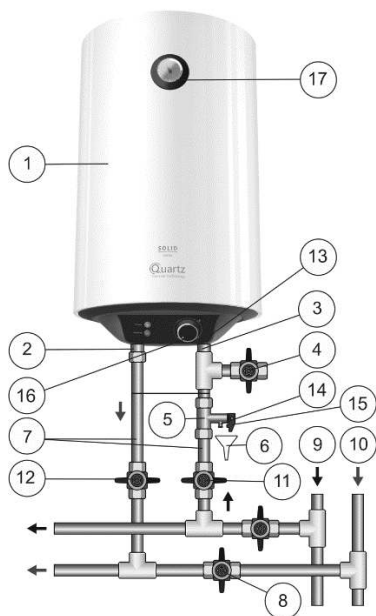
Малюнок 1. Схема підключення ЕВН до водопроводу
