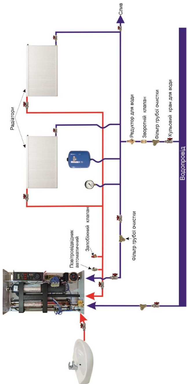
Мал.1. Рекомендована схема опалення DUOS 6,9,12,15 кВт
