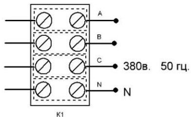
Мал.5 Схема підключення котла до мережі 380в
