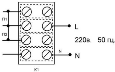
Мал.4 Схема підключення котла до мережі 220в
