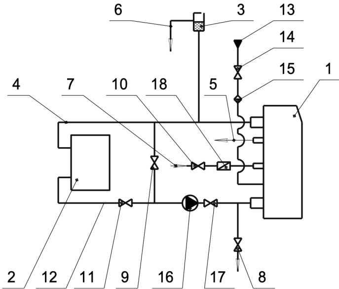
Мал. 2.3 - Схема підключення апарату до опалювальної системи з примусовою циркуляцією теплоносія.
