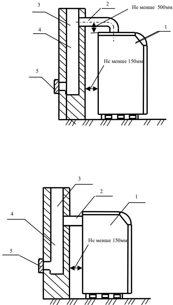
Рис.2.1 Схема встановлення апарата 1-апарат; 2-з'єднувальний патрубок ; 3-димохід; 4- кишеня; 5- дверці для чистки димохода.
