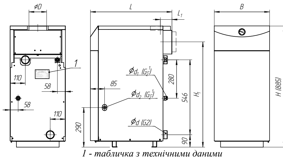
Рисунок 1 Приєднувальні розміри котлів
