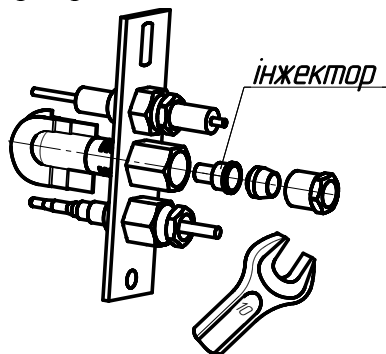
Рис.7 Заміна інжектора пілотної пальника
