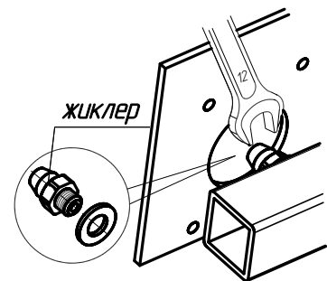
Рис.6 Заміна жиклерів основного пальника
