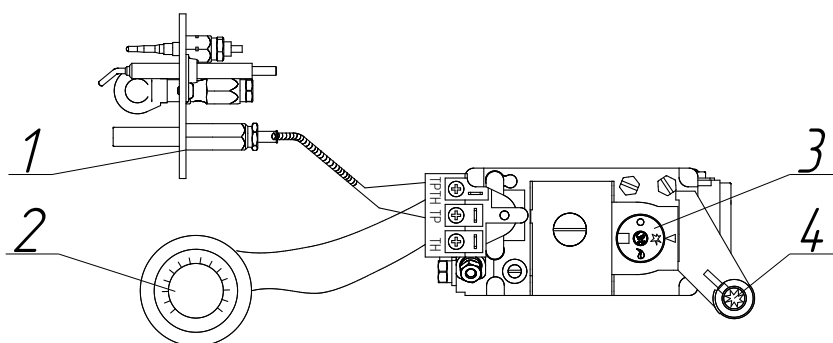
Рисунок 4 Котел газовий опалювальний сталевий "Данко – 20CH...28CH"
