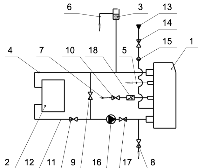
Рис. 4 - Схема підключення апарату до опалювальної системи закритого типу з примусовою циркуляцією теплоносія.
