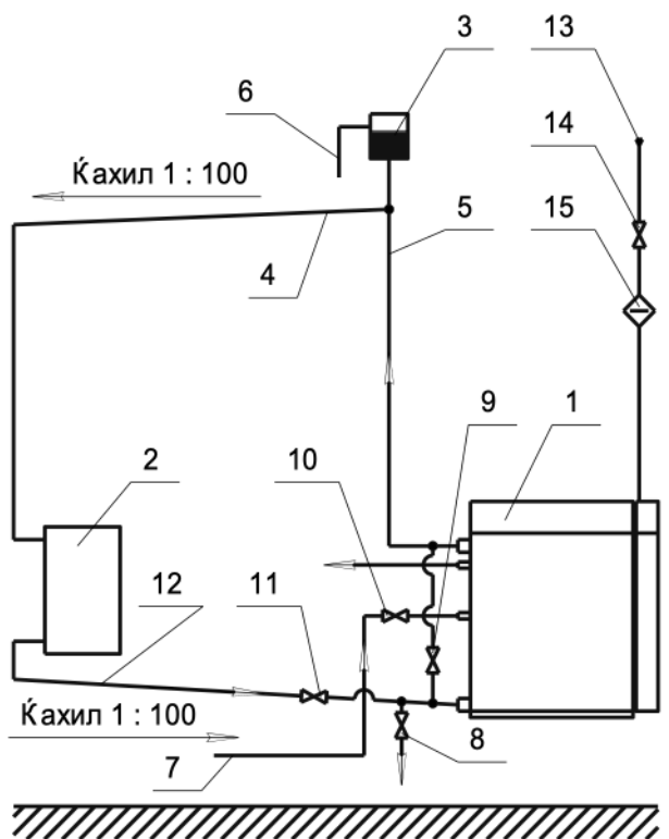
Рис. 3 - Схема підключення апарату до опалювальної системи відкритого типу з природною циркуляцією теплоносія
