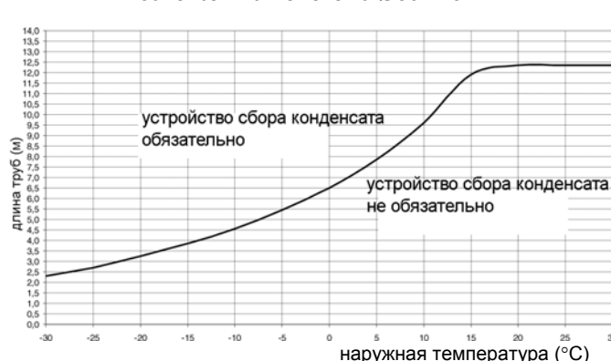
Коаксиальная система Ø80/125 мм
