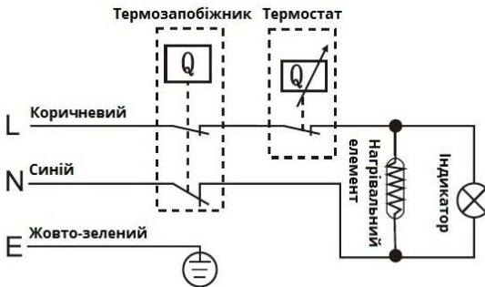
Електрична схема водонагрівача:
