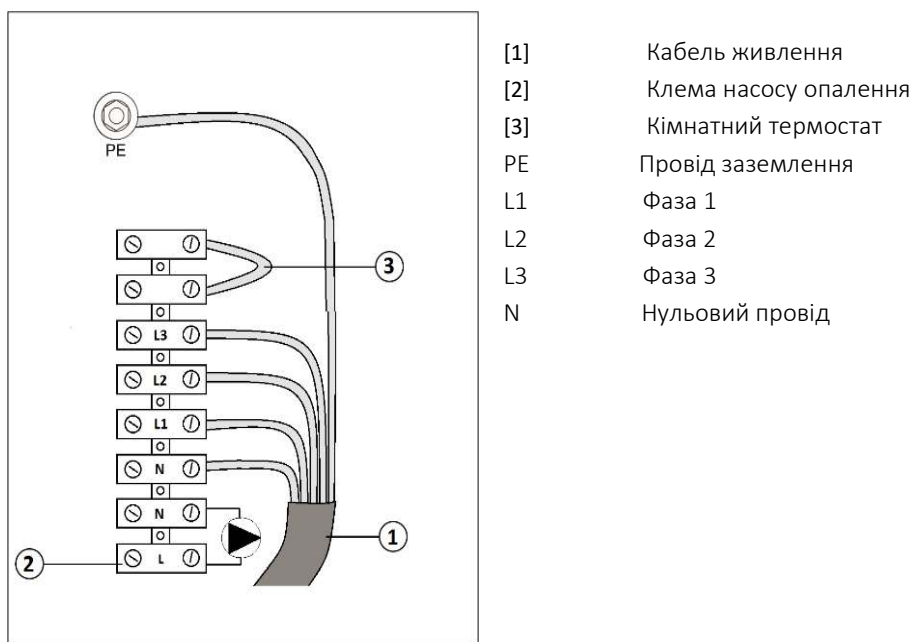
Рис. 7 Підключення до електромережі 380 В 3–9 кВт, 3х 400/230 В AC
