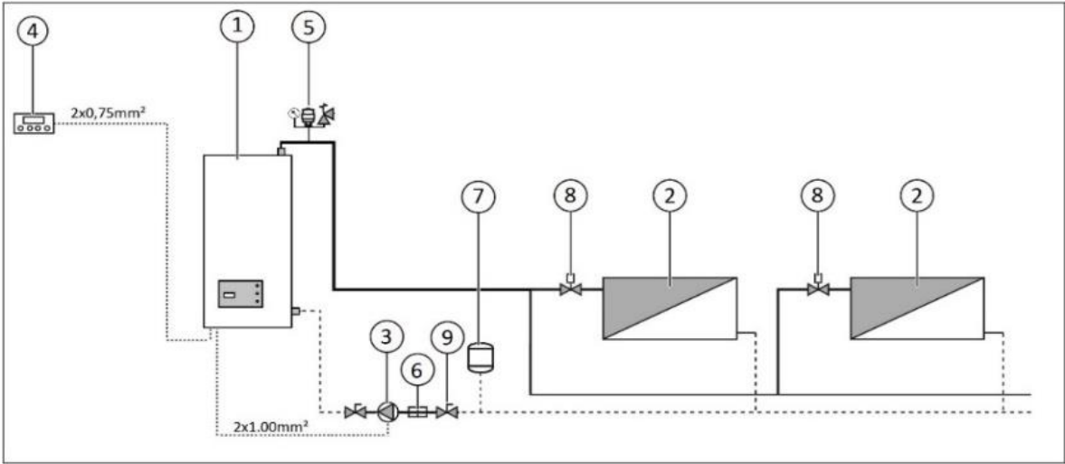
Рис. 10 Режим опалення та нагрівання гарячої води в баку непрямого нагріву
