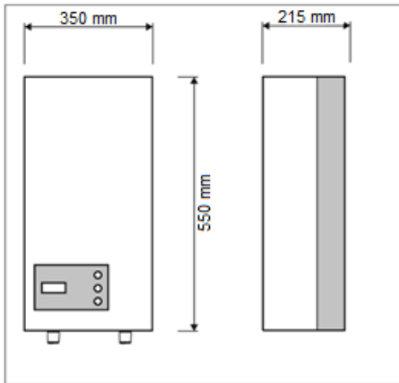
Рис. 2 Розміри опалювального котла AVL Joule A JX-SPT
