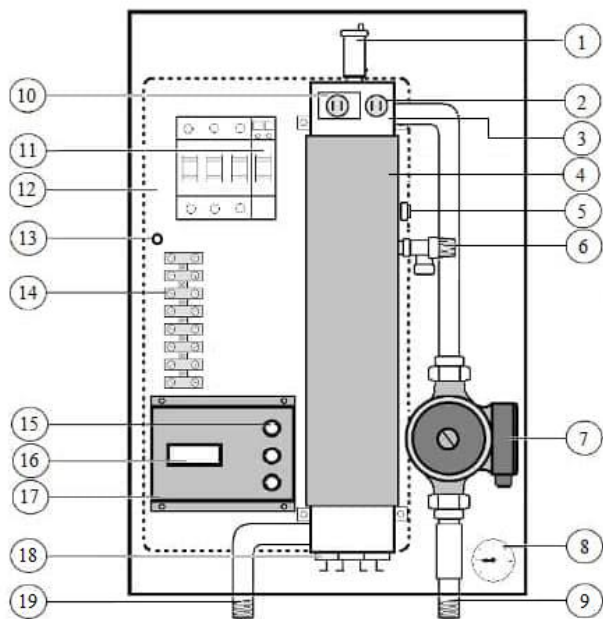
Рис. 1 Функціональні елементи котла AVL Joule A JX-SPT 4.5-9 кВт
