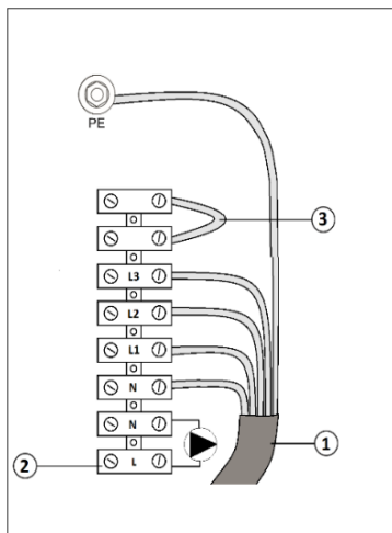
Рис. 6 Підключення до електромережі 380 В 4,5-12 кВт, 3x 400/230 В АС
