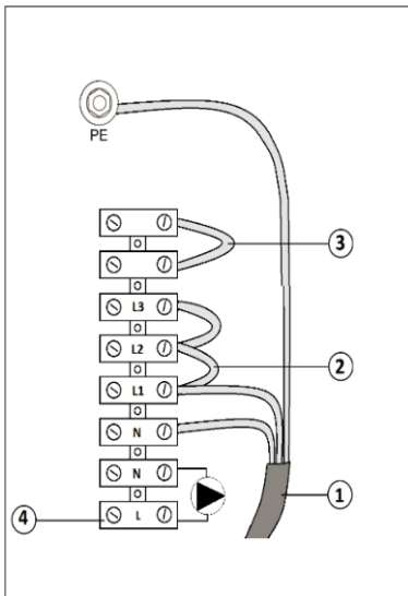
Рис. 5 Підключення до електромережі 4,5-9 кВт, 1x230 В АС
