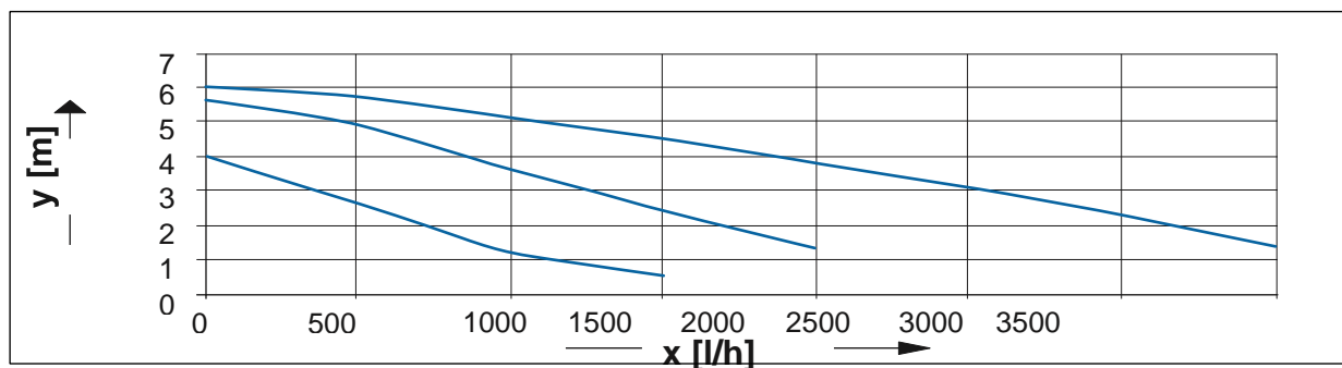
Рис. 8 Напір насоса на прикладі Wilo RS15/6
