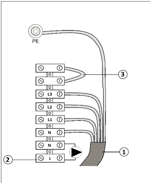
Рис. 13 Подключение к электросети 380 В 4.5-12 кВт, 3x 400/230 В AC
