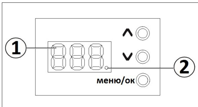
Рис. 14 Панель управления отопительного котла AVL Joule AJX-SPT eco
