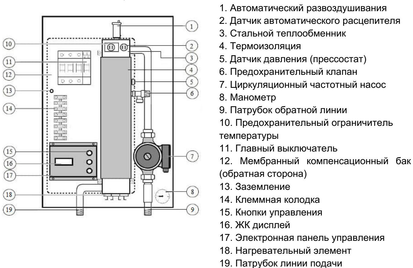
Рис. 1 Функциональные элементы котла AVL Joule AJX-SPT eco
