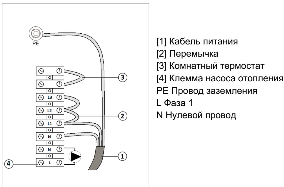
Рис. 12 Подключение к электросети 4.5-9 кВт, 1x230 В AC
