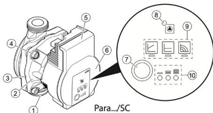
Рис. 4 Циркуляционный насос Wilo-Para SC
