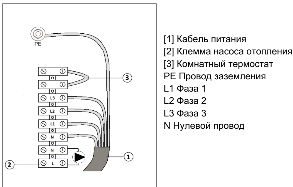
Рис. 13 Подключение к электросети 380 В 4.5-12 кВт, 3х 400/230 В AC
