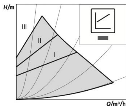
Рис. 15 Переменный перепад давления \Delta p_v (I, II, III)
