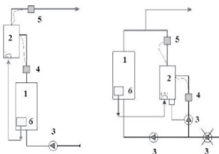
А Мал. 4 - Комбіноване опалення. Схеми підключення електродкотла
