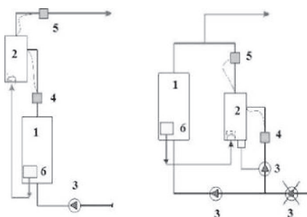
А - послідовне підключення до системи; Б - паралельне підключення до системи; 1 - газопальний котел 2 - електричний котел 3 - циркуляційний насос 4 - датчик зворотного трубопроводу електричного котла 5 - датчик прямого трубопроводу електричного котла 6 - система управління газопальним котлом
