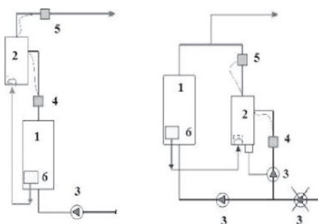
А Б Мал. 4 - Комбіноване опалення. Схеми підключення електродкотла
