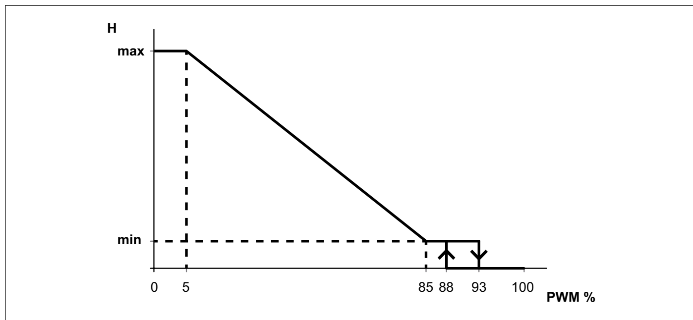
Рис. 27 Сигнал ШІМ
