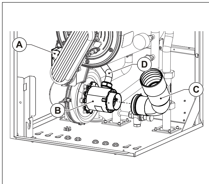
Рис. 34 Забірна труба
