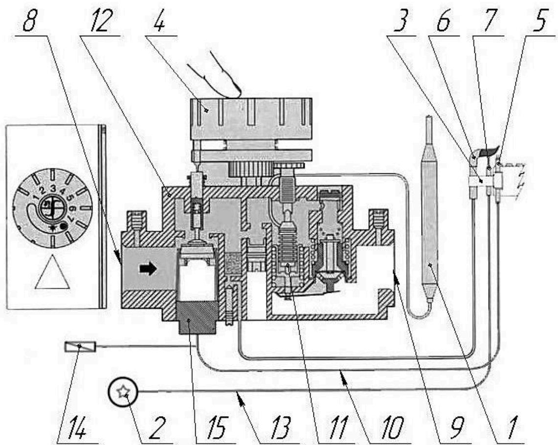
Рисунок 3 – Блок управління
