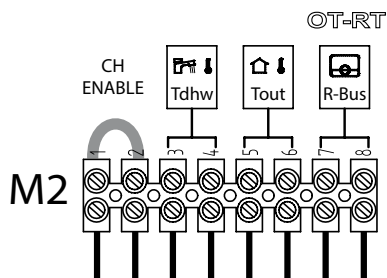
Рис. 32 Підключення кімнатного термостата (OT) або (R-Bus)
