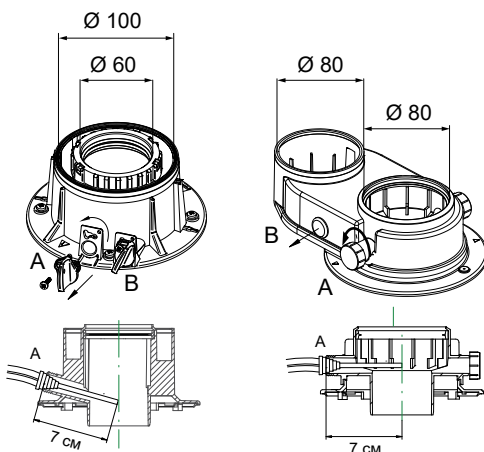
Рис. 41 Тип адаптера димоходу – точка вимірювання димових газів
