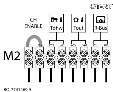
Рис. 32 Підключення кімнатного термостата (OT) або (R-Bus)
