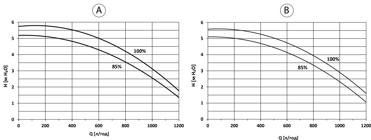
Рис. 9 Графік, що показує залежність залишкового тиску нагнітання насоса від витрати води
