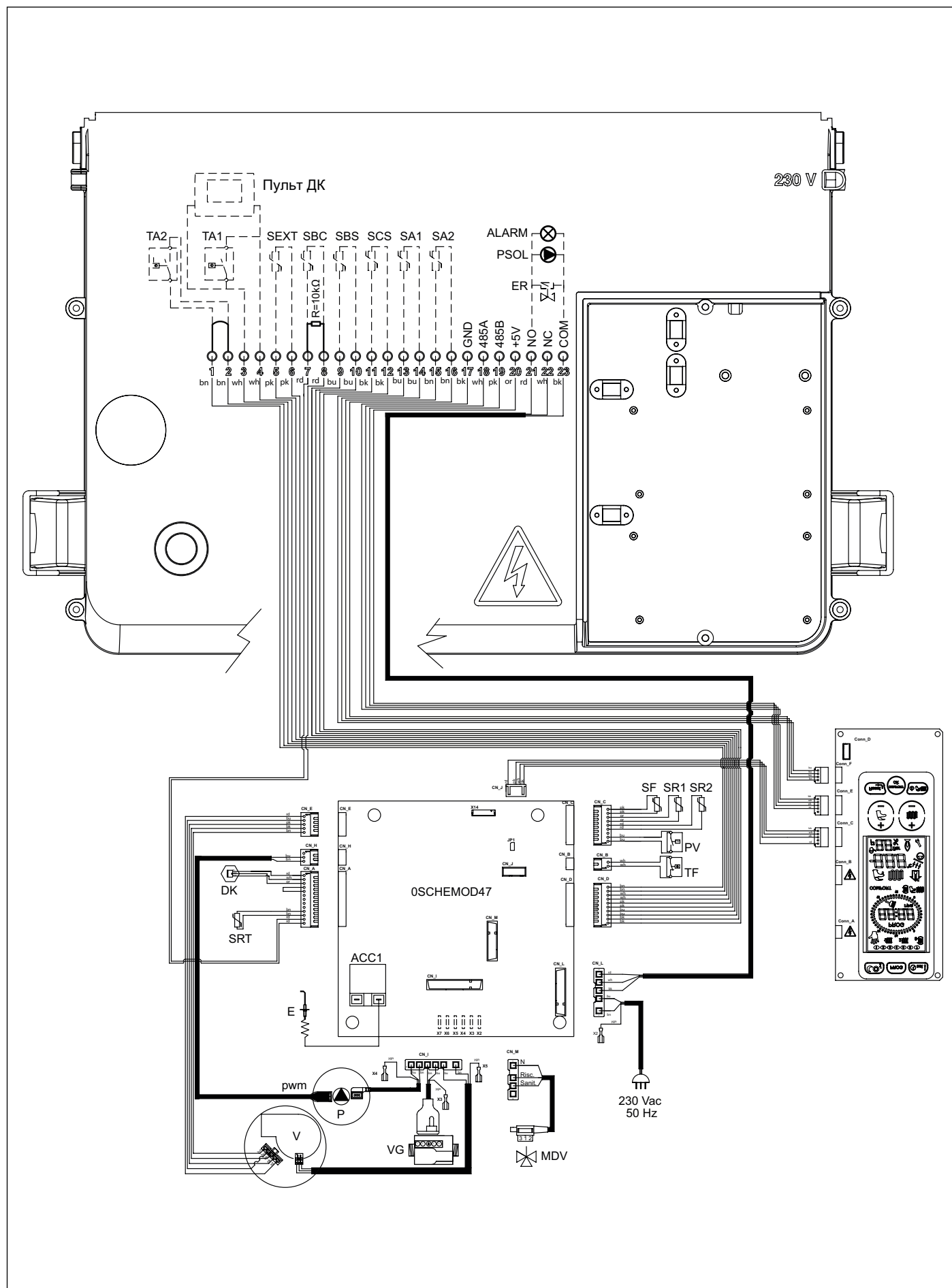
Рис. 32 Електрична схема KRB
