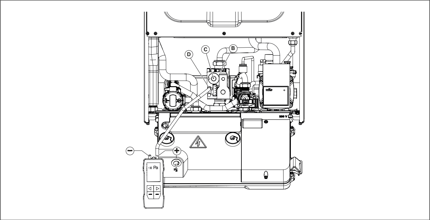
Рис. 41 Регулювання протитиску
