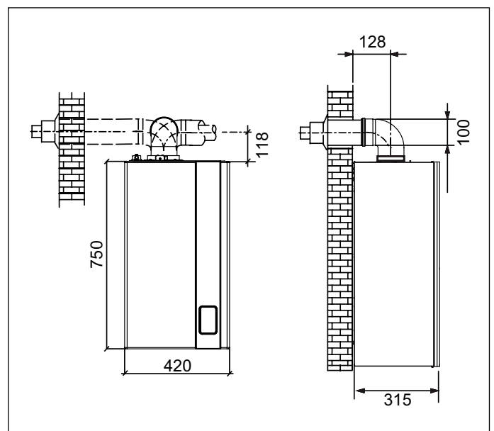
Рис. 12 Відстань між каналами забору повітря та димовиведення типу С33
