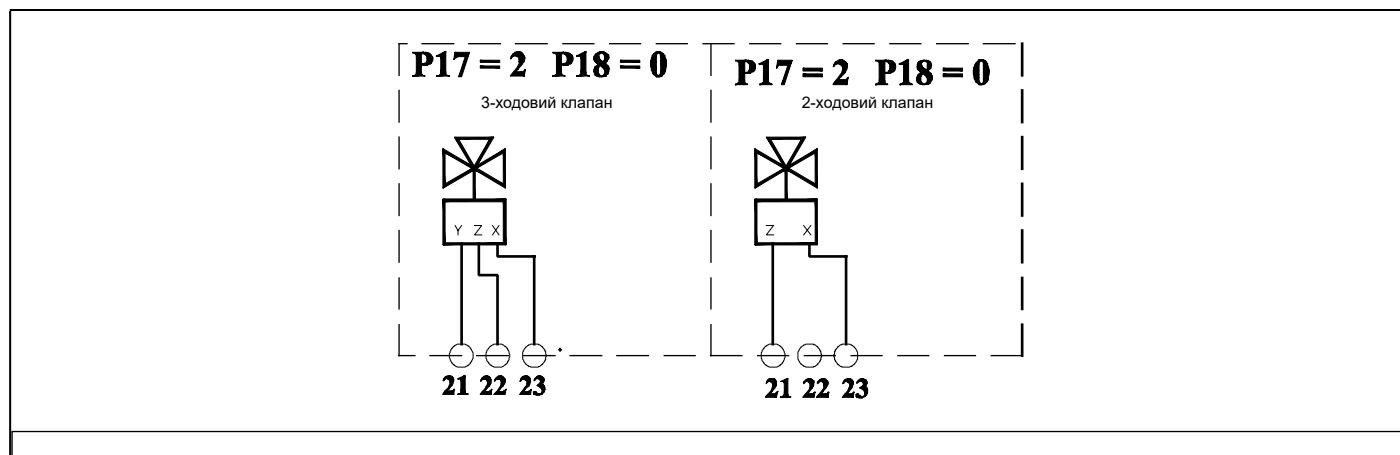
Рис. 28 Схема підключення багатофункційного реле (X = загальний; Y = на котел; Z = на колектор)
