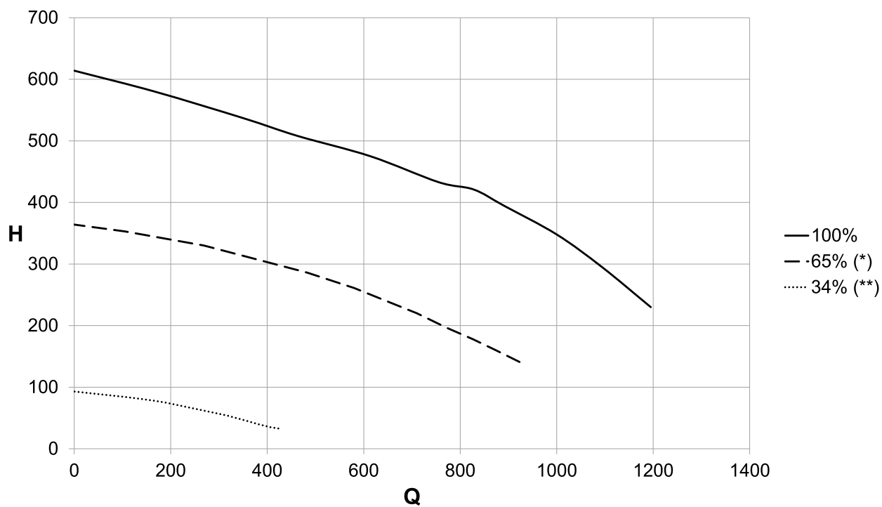
Рис. 22 Наявний напір KC-KR-KRB 28
