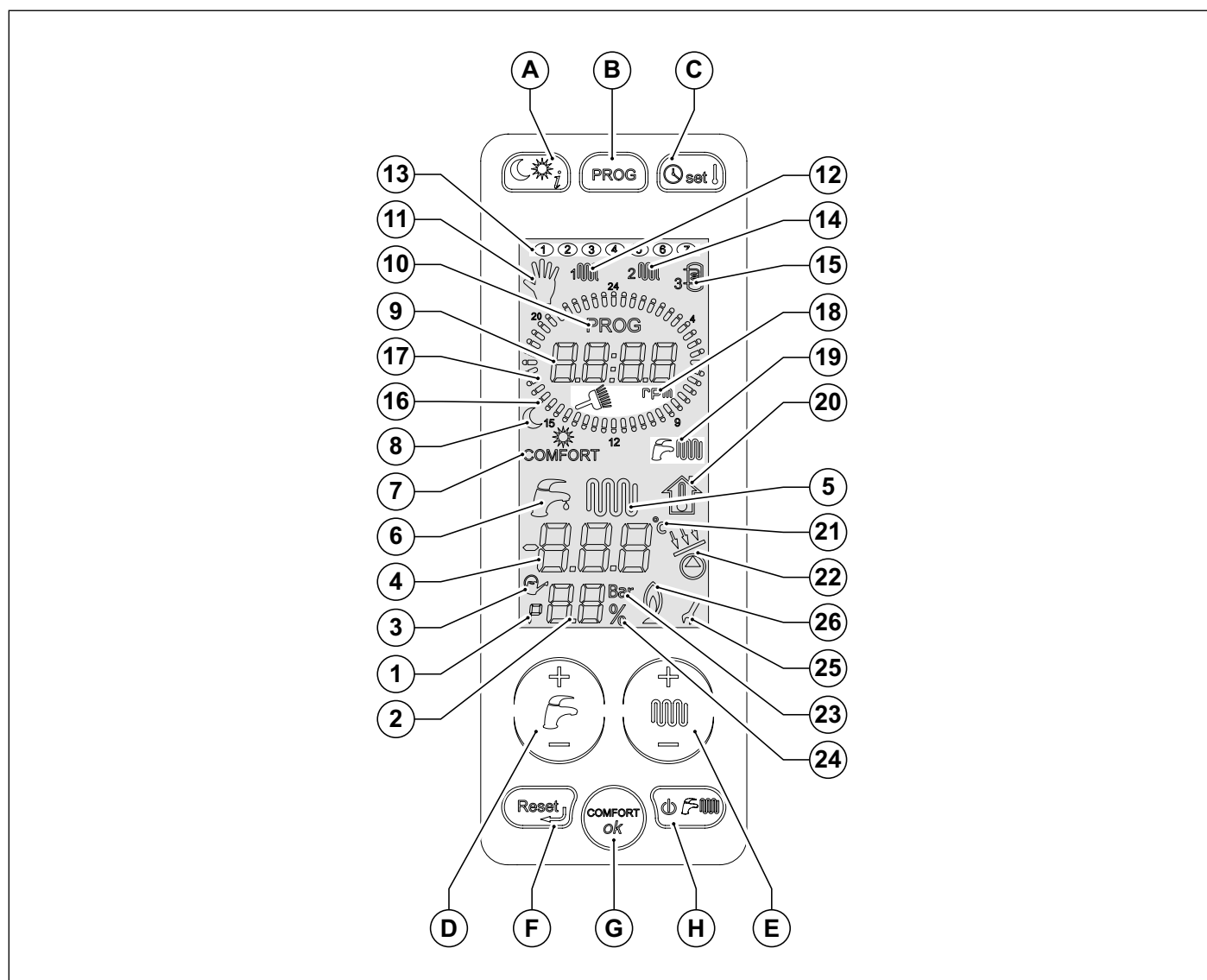
Рис. 1 Панель керування
