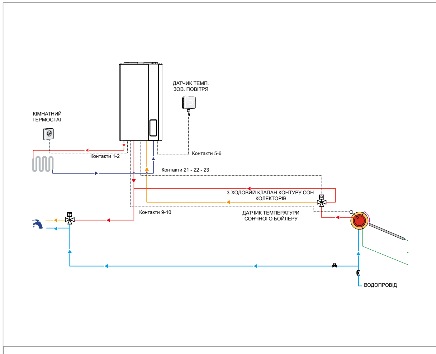
Рис. 27 Схема підключення системи сонячних коелкторів з природнею циркуляцією до двохконтурного котла
