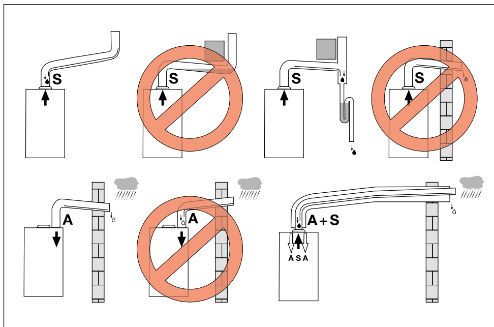
Рис. 10 Приклади монтажу
