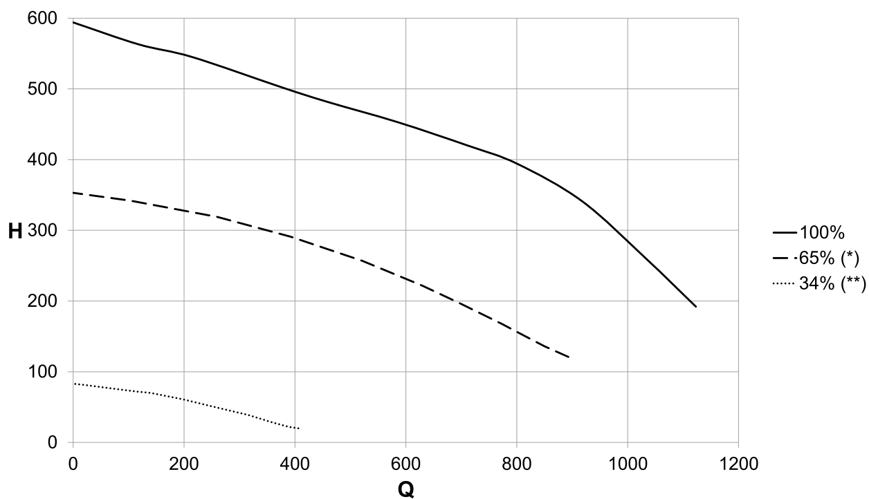
Рис. 21 Наявний напір KC-KR-KRB 24
