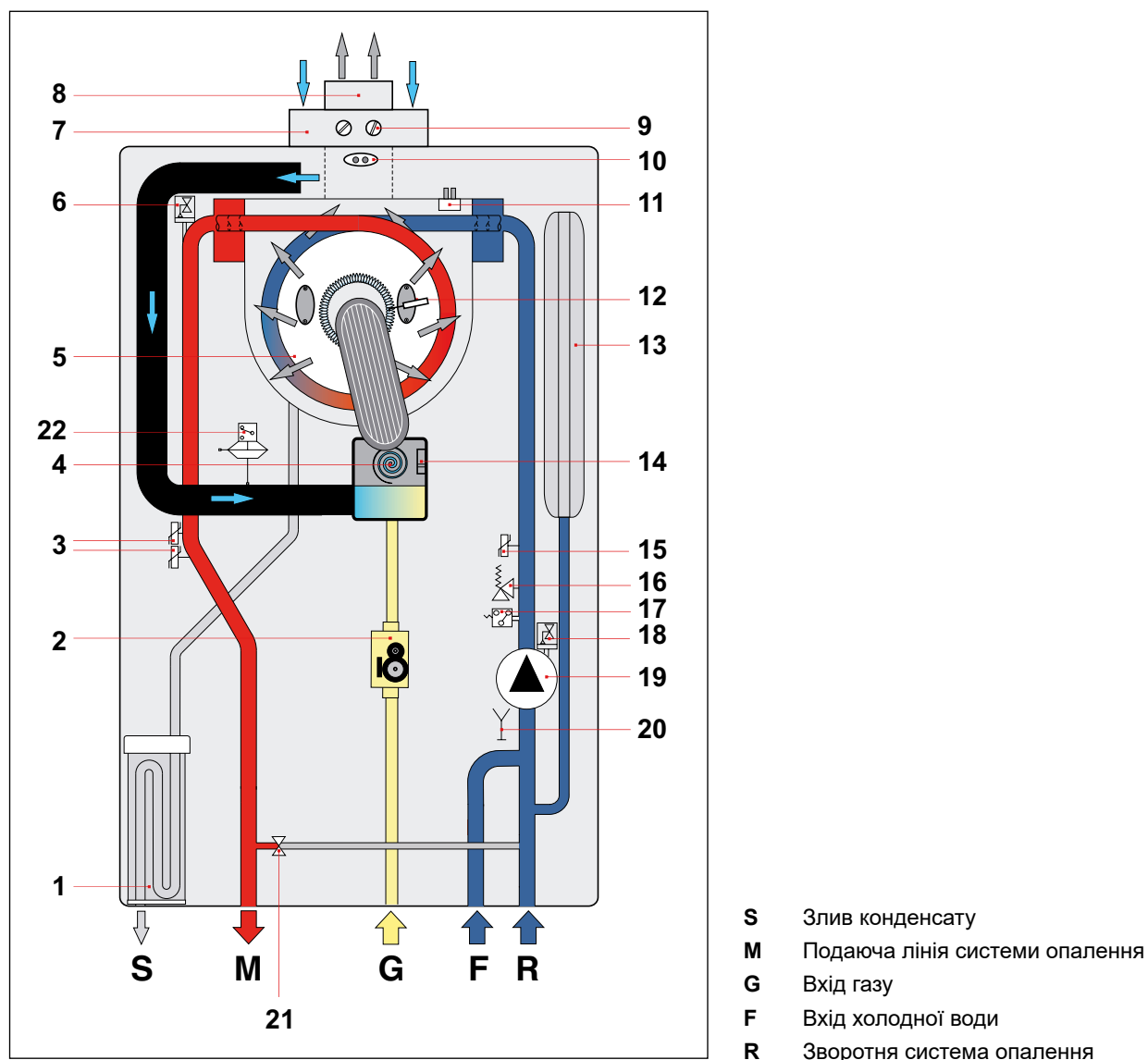
Рис. 7 Гідравлічна схема моделі KR
