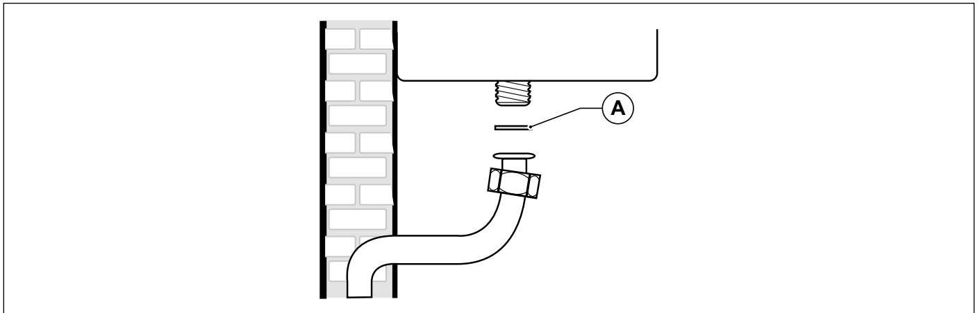
Рис. 17 Підключення газу
