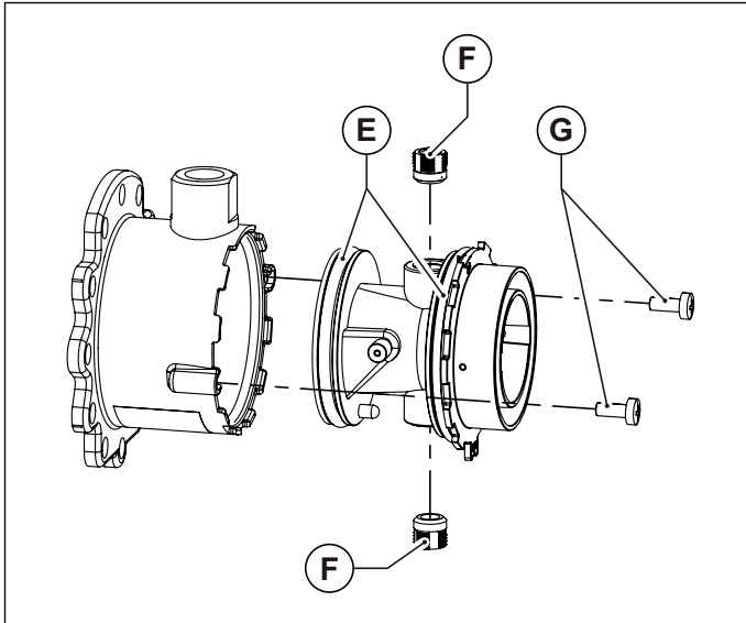
Рис. 28 Пластмасовий корпус змішувача
