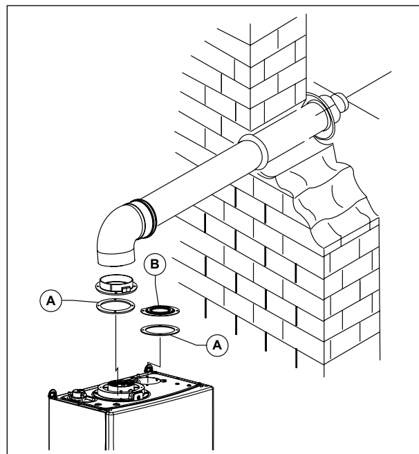
Рис. 11 Коаксиальні димоходи типу C13 - C33
