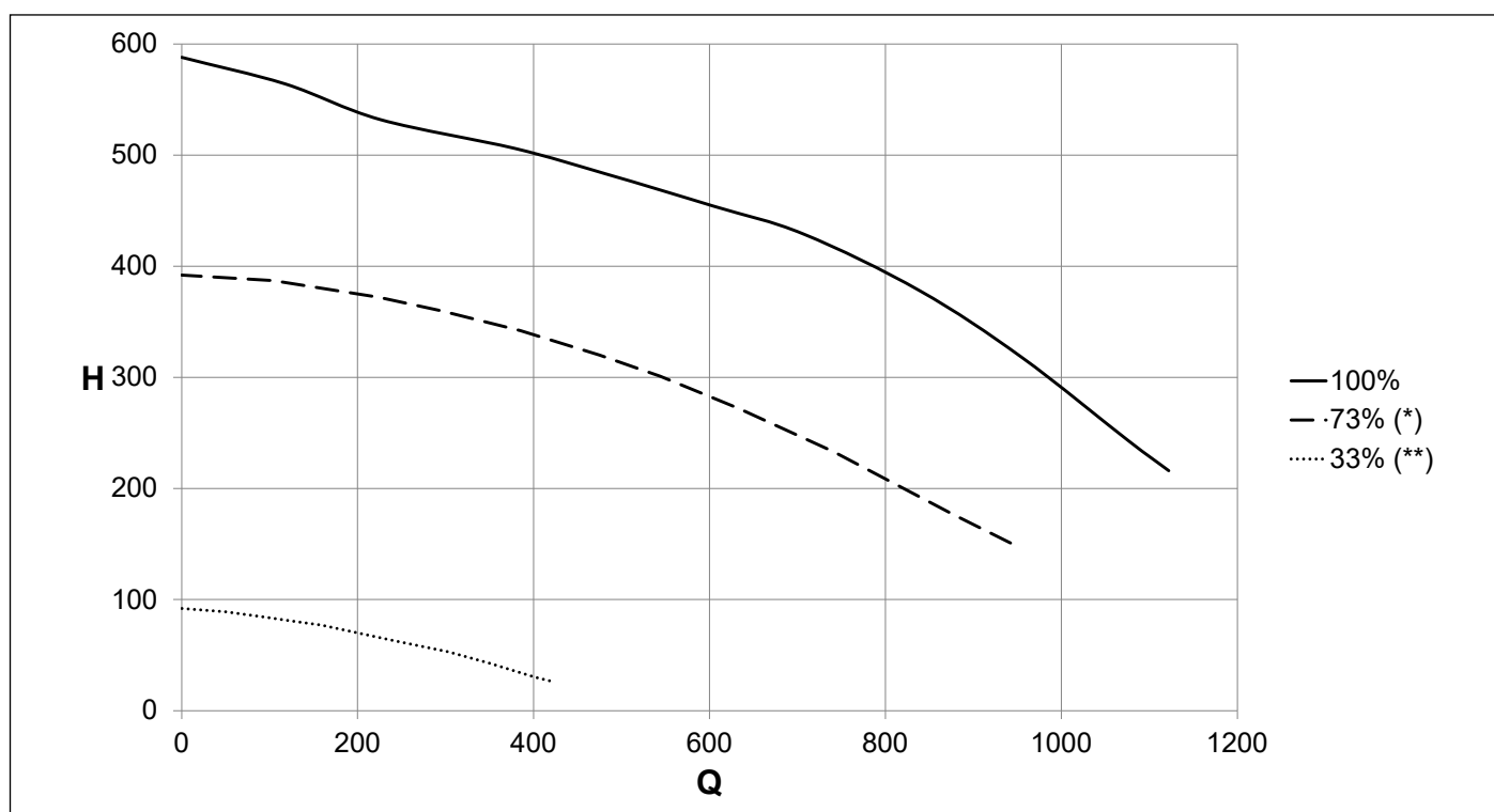
Рис. 22 Наявний напір KC-KR-KRB 28
