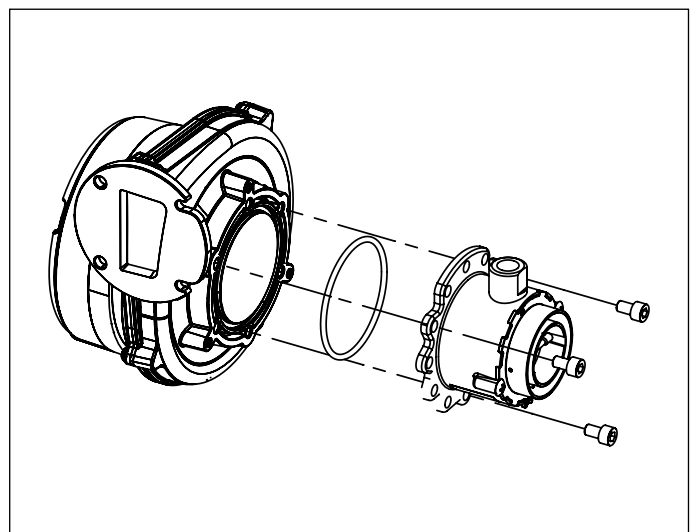
Рис. 27 Змішувач
