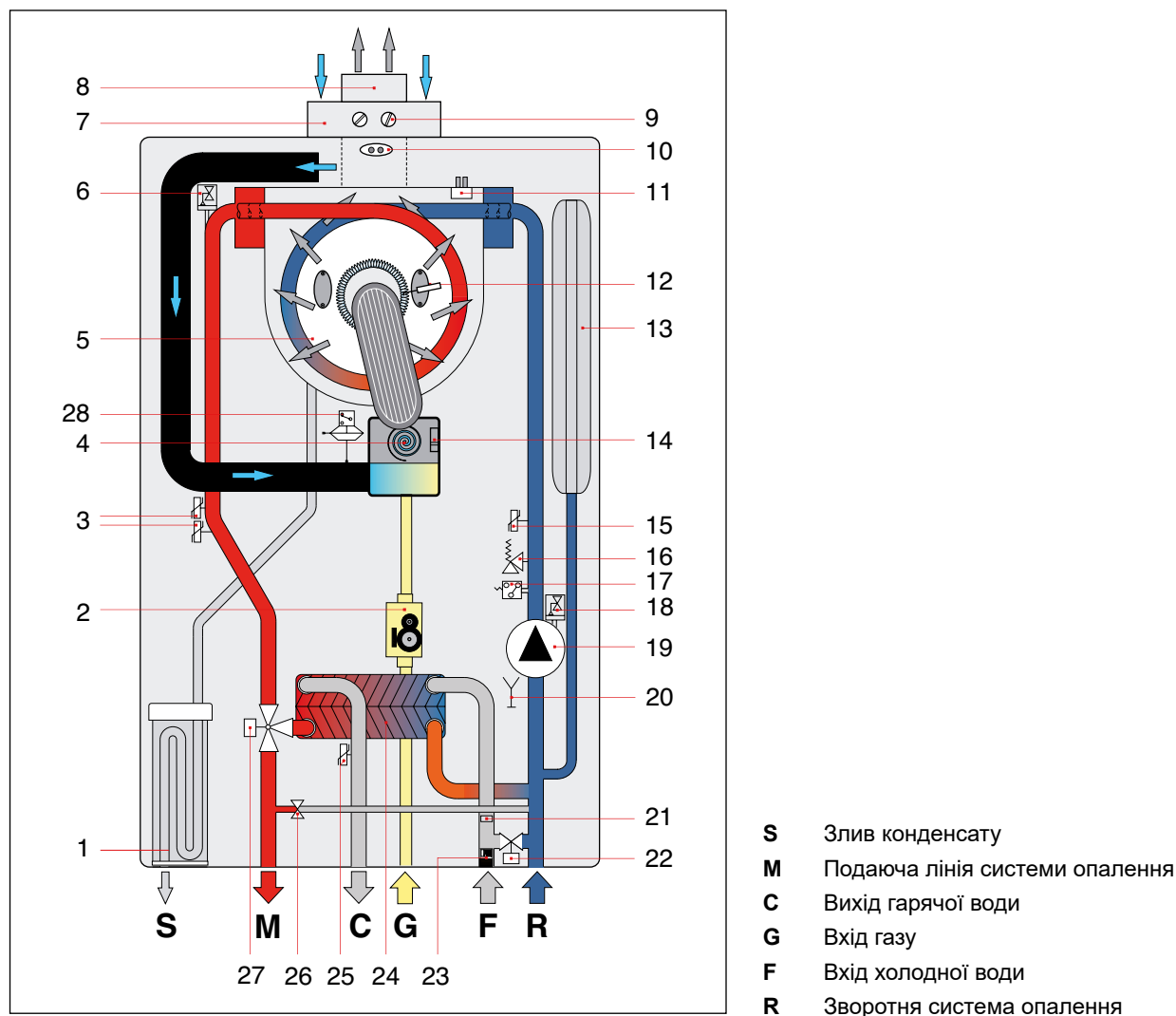
Рис. 6 Гідравлічна схема КС
