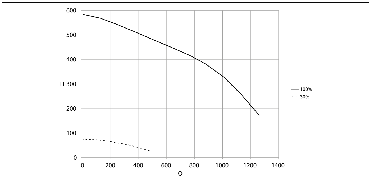
Рис. 10 Наявний напір
