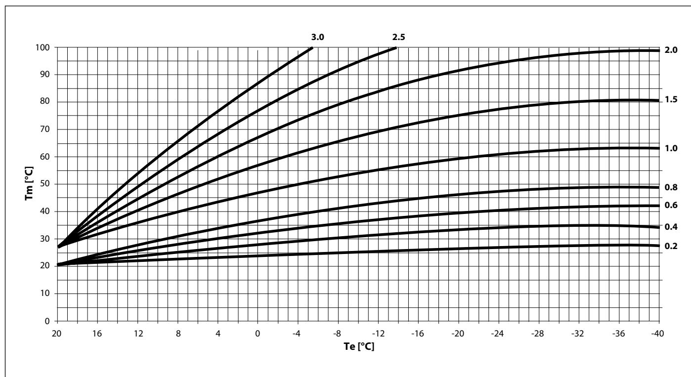
Рис. 9 Температурні криві
