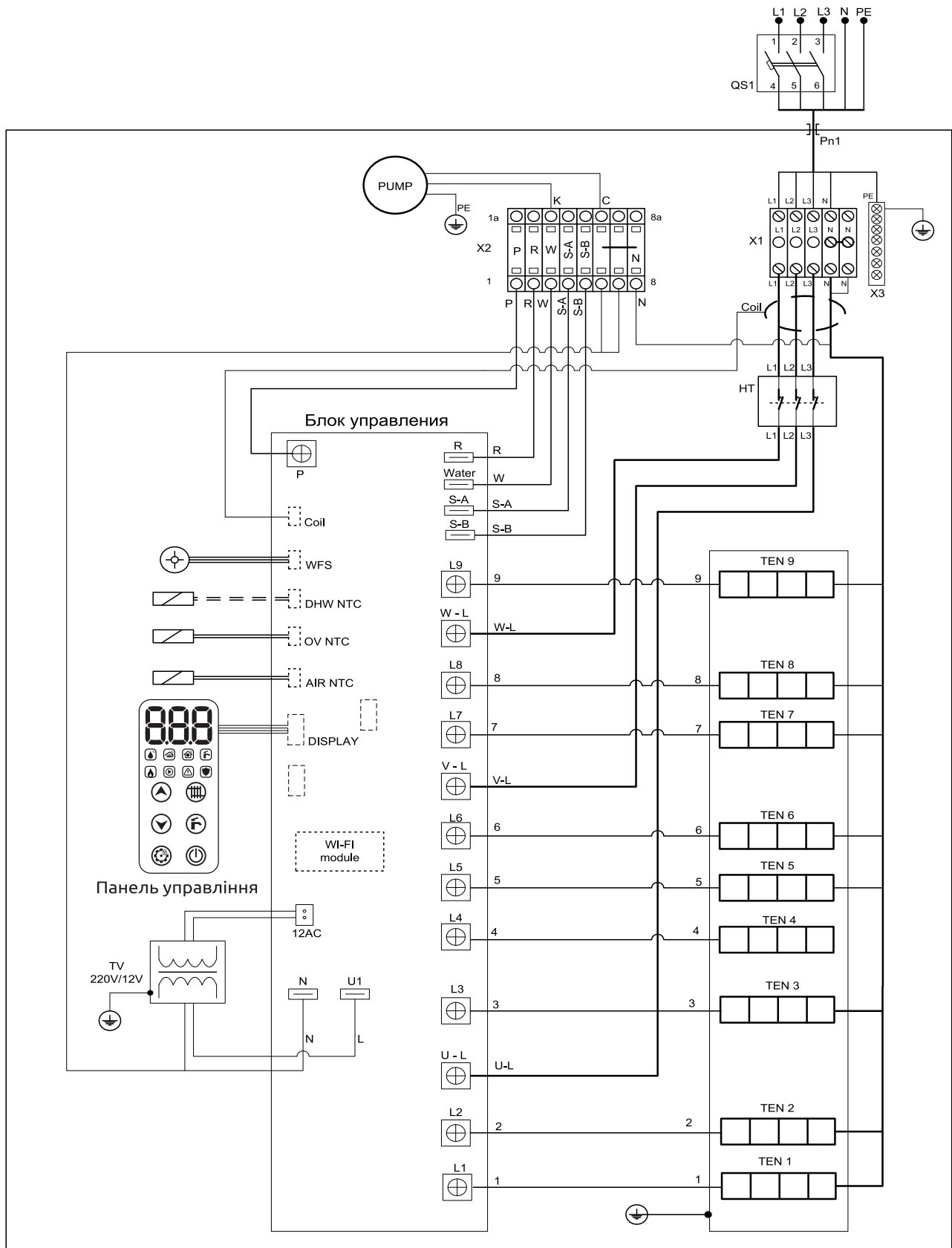
Малюнок 15 – Схема підключення котлів ESPRO 21 кВт і 24 кВт до трифазної мережі 380В (50Гц).
