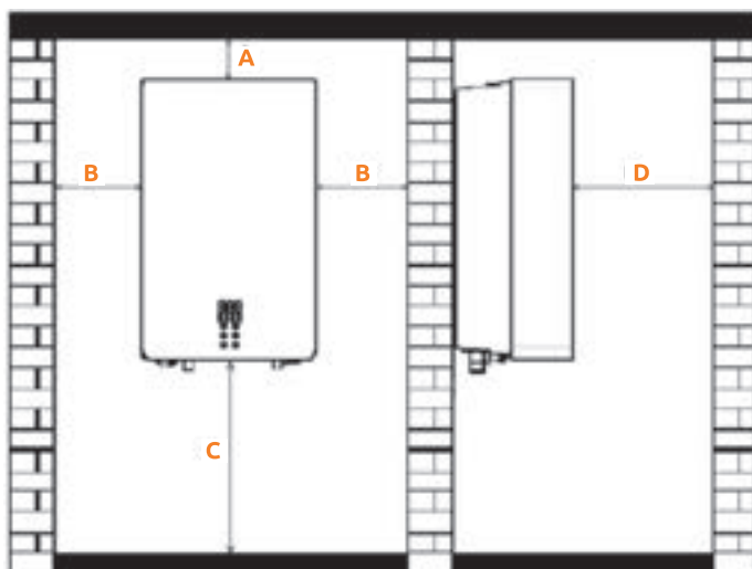
Малюнок 4 - Мінімальні вільні відстані від поверхонь до корпусу котла
