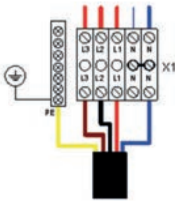
а) 3L + N + PE
