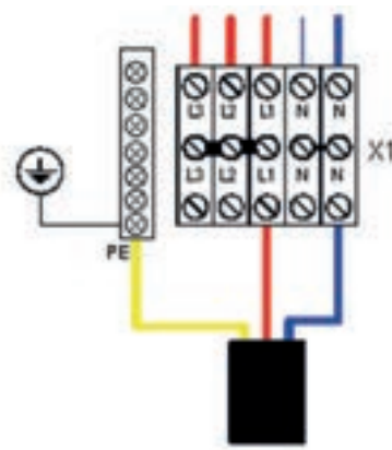
б) (L + N + PE)
