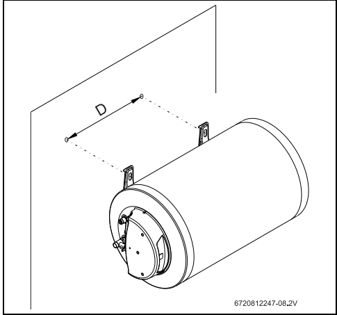
Мал. 8 Горизонтальна установка (настінний монтаж)
