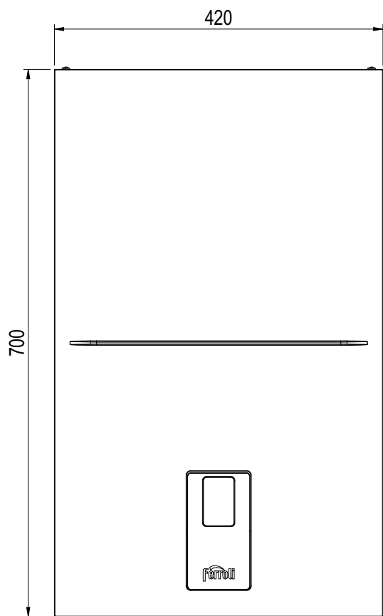
рис. 58- Вид спереди
