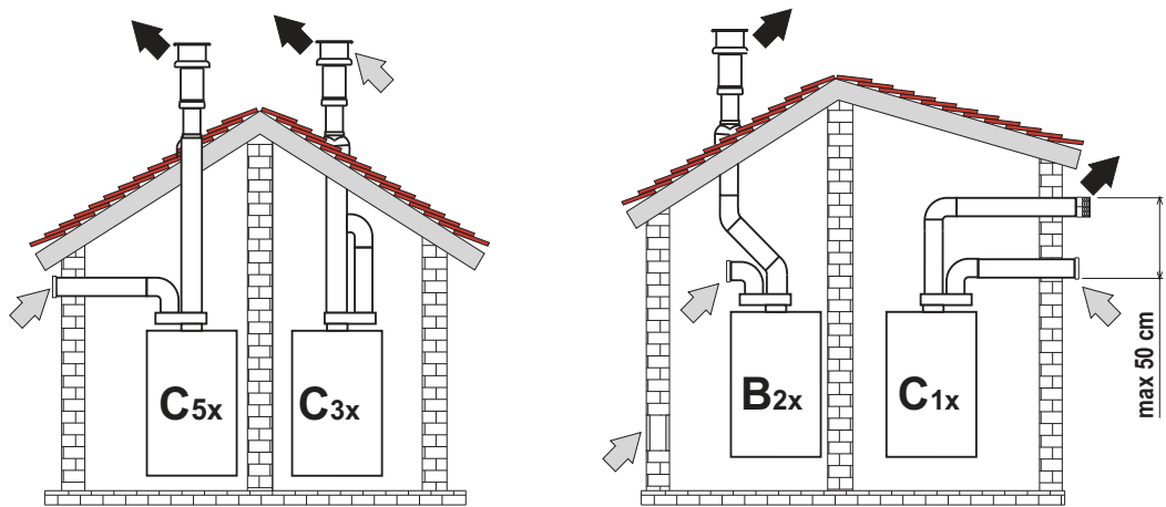
рис. 32- Примеры подсоединения с помощью раздельных труб (⇨ = Воздух/ ⇨ = Дымовые газы)
