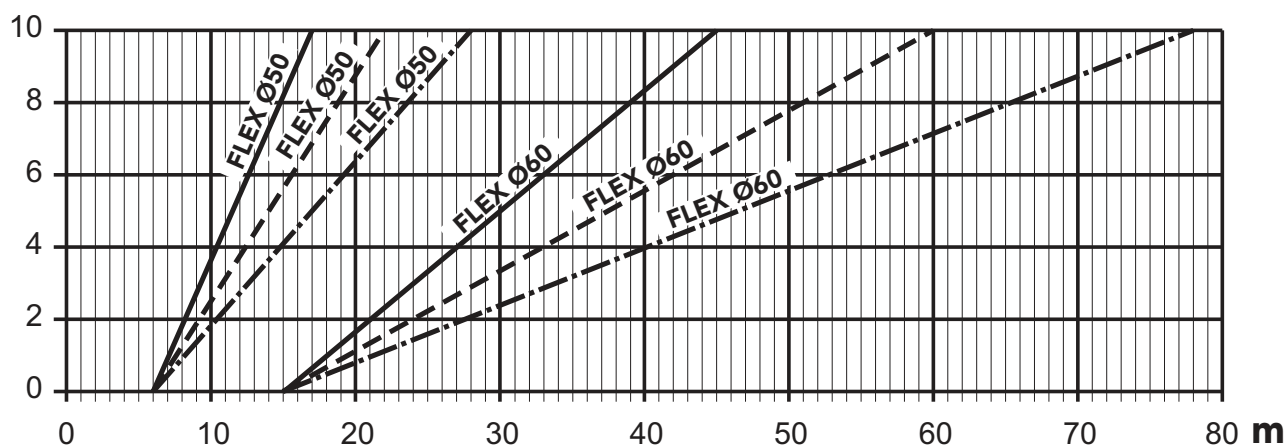
рис. 35- График выбора параметров дымохода
