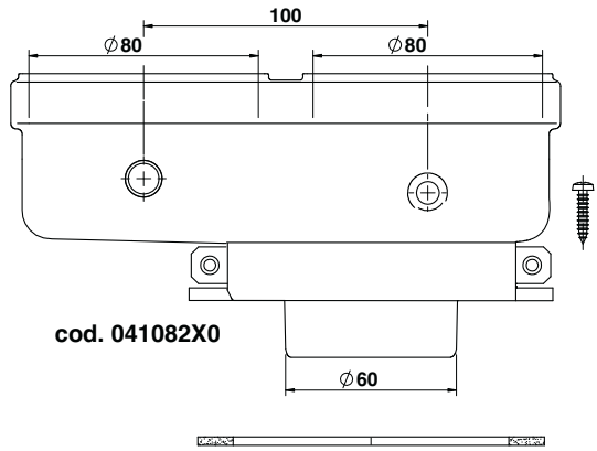
рис. 33- Исходная принадлежность для раздельных труб
