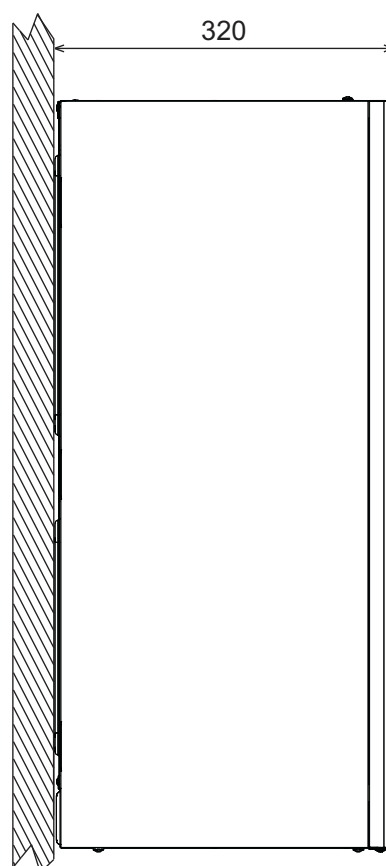
рис. 59- Вид сбоку
