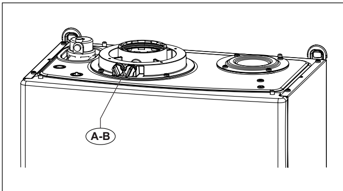
Рис. 15 Положення заглушок
