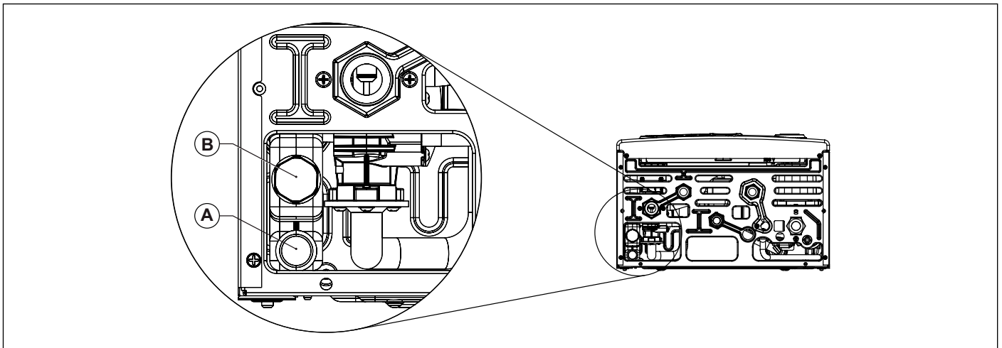
Рис. 18 Злив конденсату
