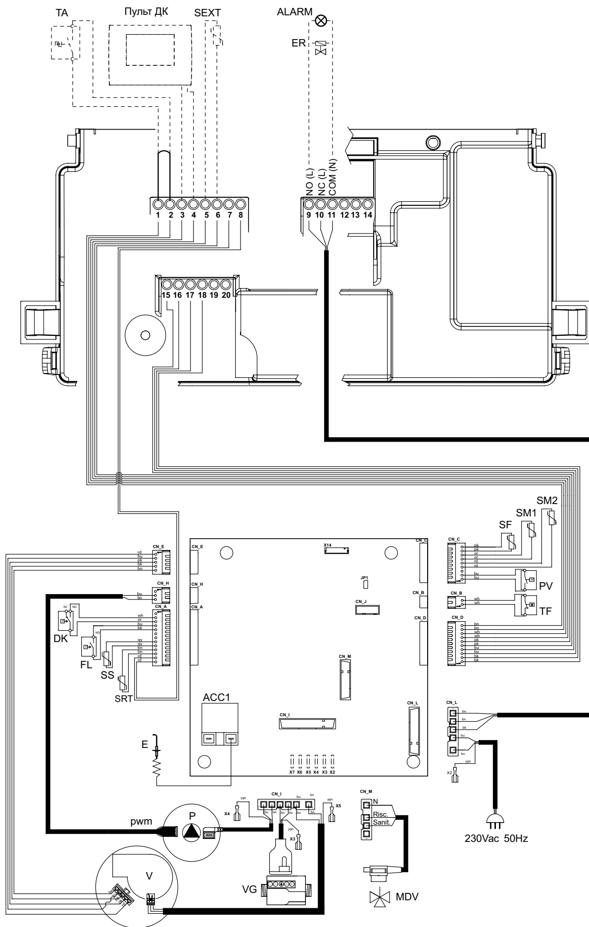
Рис. 23 Електрична схема КС
