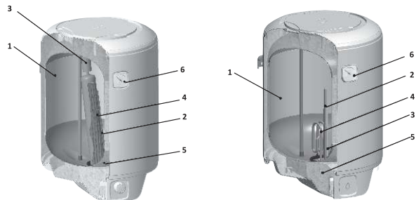
Рисунок 1. ЕВАД Atlantic в розрізі та його складові частини:
