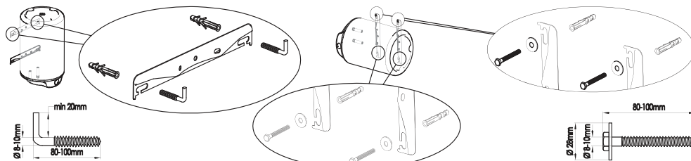
Рисунок 4. Кріплення ЕВАД до стіни
