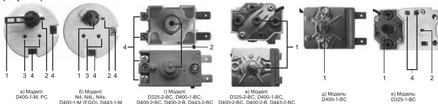
1 – Регулятор температури; 2 – Кнопка теплового захисту; 3 – Гнізда підключення сигнальної лампи; 4 – Клемми підключення до електромережі
