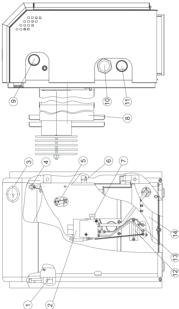
Рис. 1. Устройство котла
