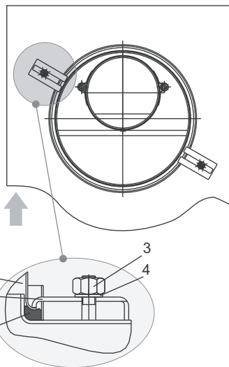
Рис. 4. Схема крепления воздуховода 1 - воздуховод; 2 - шнур базальтовый теплоизоляционный; 3 - гайка; 4 - шайба; 5 - прижим
