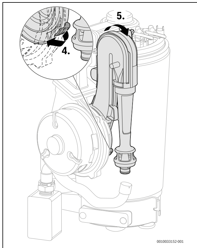
Мал. 49 Знімання трубки Вентурі
