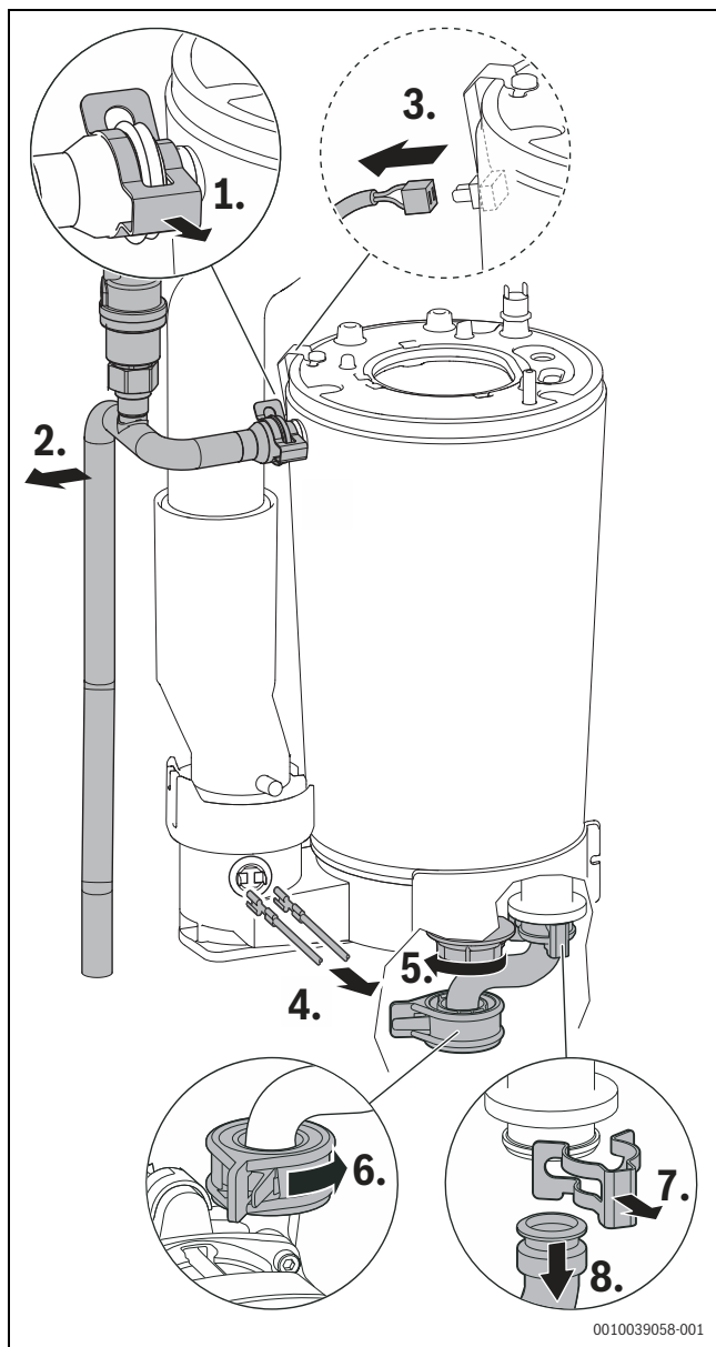
Мал. 63 Від'єднання труби лінії подачі, зняття кабелю та зняття труби зворотної лінії
