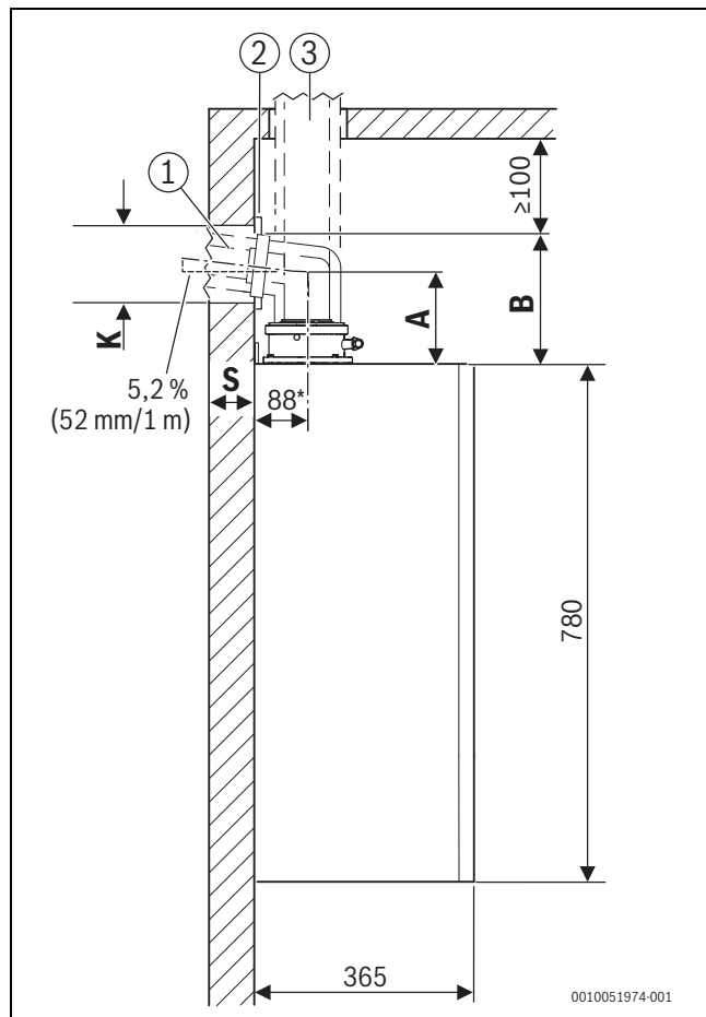
Мал. 2 Вигляд збоку (мм)
