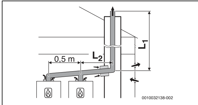
Мал. 23 Каскад з 2 приладами: система відведення димових газів у шахті із жорсткою конструкцією відповідно до B 53p з подачею повітря у прилад з приміщення
