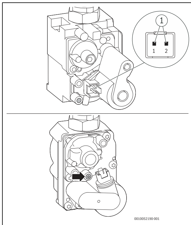
Мал. 47 Точки вимірювання на газовій арматурі
