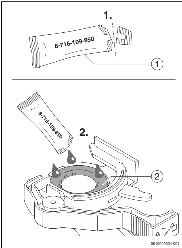
Мал. 81 Змащення ущільнення
