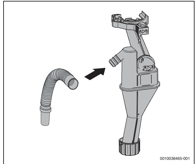
Мал. 32 Встановлення шланга для відведення конденсату на штуцер
