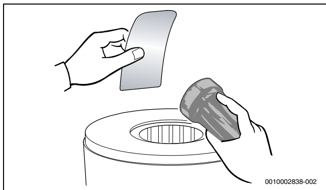
Мал. 61 Перевірка котлового блоку, який включає камеру згоряння і теплообмінник, на наявність відкладень
