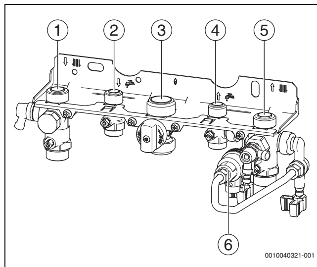
Мал. 35 Підключення газопроводів та трубопроводів подачі води
