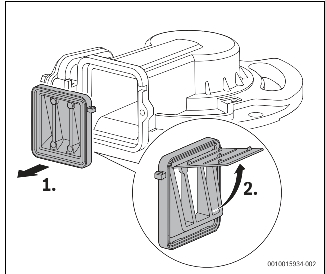
Мал. 53 Захист від зворотного потоку в змішувальному пристрої
