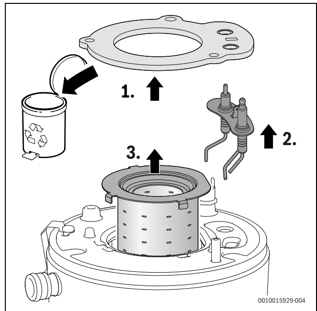
Мал. 54 Виймання пальника
