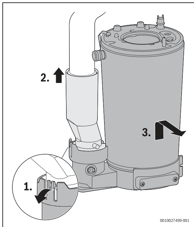
Мал. 64 Демонтаж котлового блока, який включає камеру згоряння і теплообмінник
