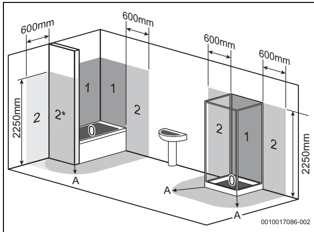
Мал. 25 Захисні зони (приклад)
