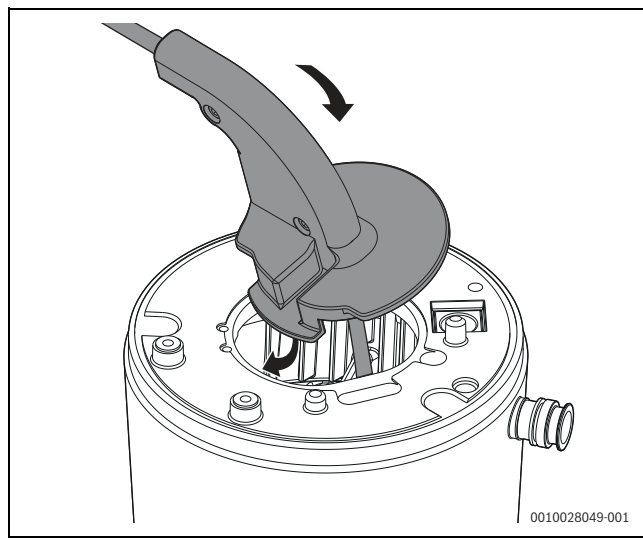
Мал. 57 Вставте щітку у котловий блок, який включає камеру згоряння і теплообмінник
