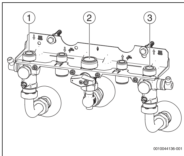
Мал. 36 Підключення газопроводів та трубопроводів подачі води
