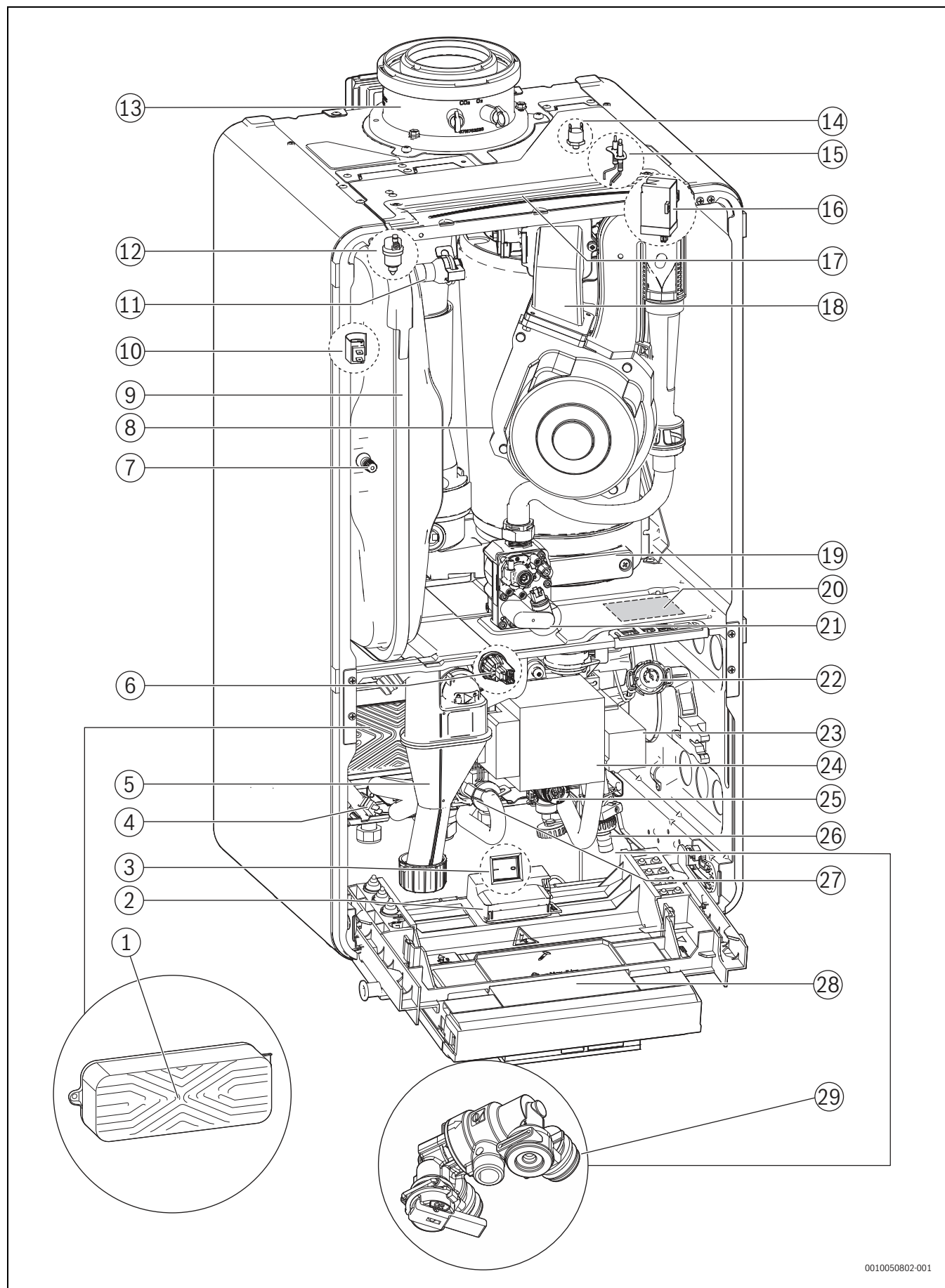
Мал. 6 Огляд виробу, двоконтурний котел
