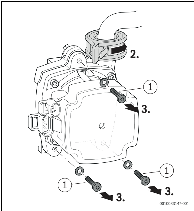
Мал. 66 Розблокуйте насос опалювального контуру та зніміть гвинти
