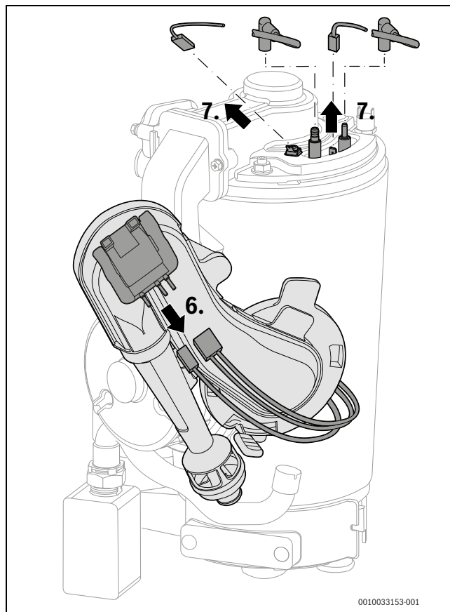
Мал. 50 Знімання кабелів
