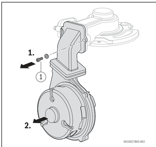
Мал. 52 Демонтаж вентилятора зі змішувальною камерою
