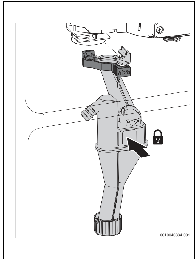
Мал. 82 Встановлення сифона для відведення конденсату
