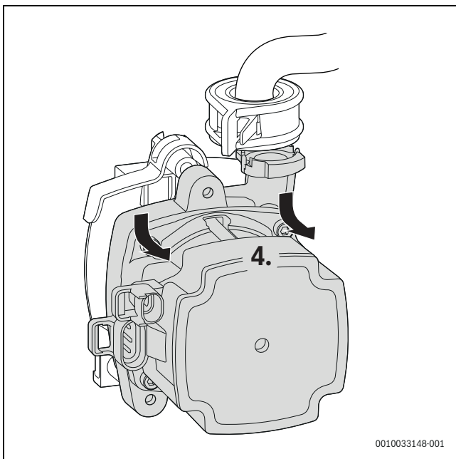
Мал. 67 Знімання насоса опалювального контуру
