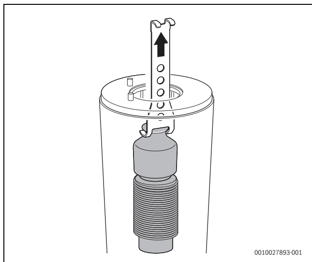
Мал. 55 Виймання верхнього елемента теплообмінника, що служить для оптимізації розподілювання тепла
