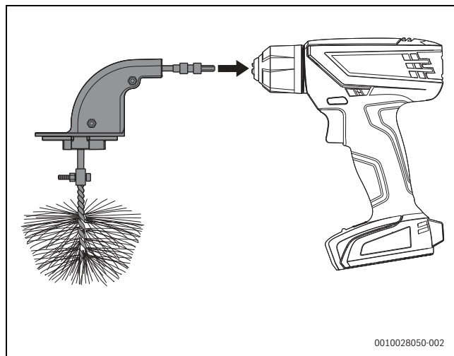
Мал. 58 З'єднайте щітку з акумуляторним шурупвертом
