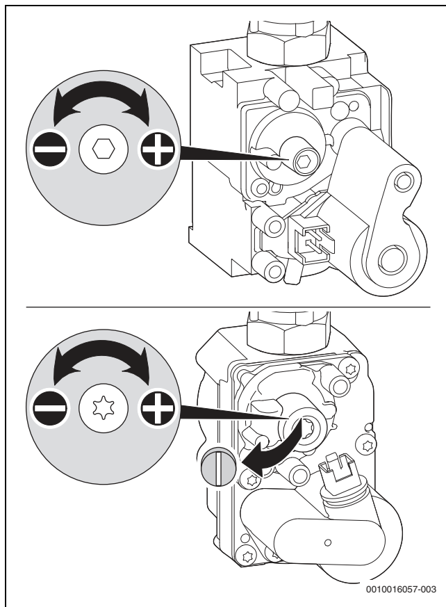
Мал. 44 Регулювання газової арматури
