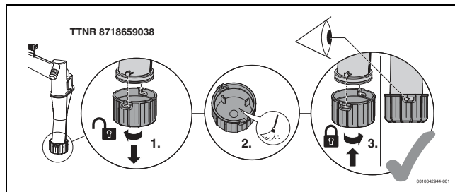
Мал. 79 Очищення брудовловлювача
