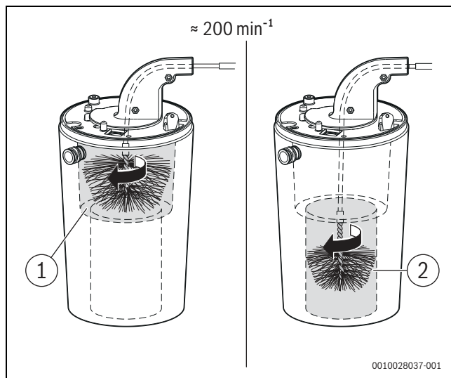
Мал. 59 Чищення котлового блоку, який включає камеру згоряння і теплообмінник (200 об/хв, тільки при правосторонньому обертанні)
