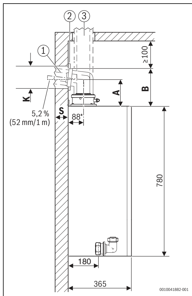
Мал. 4 Вигляд збоку (мм)
