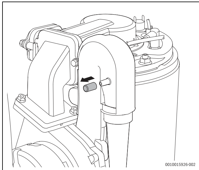
Мал. 46 Штуцер для вимірювання на змішувальній камері
