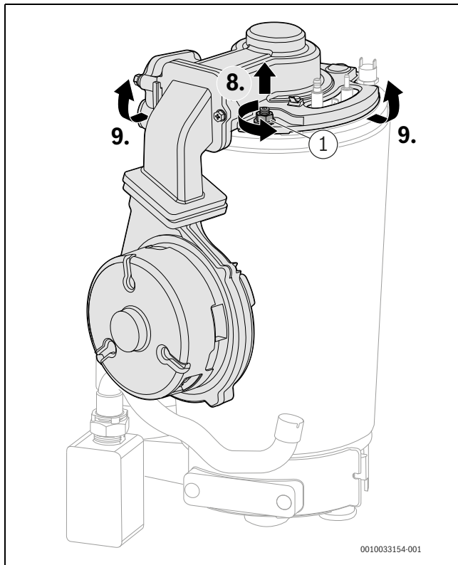
Мал. 51 Знімання кришки пальника разом з вентилятором та змішувальною камерою
