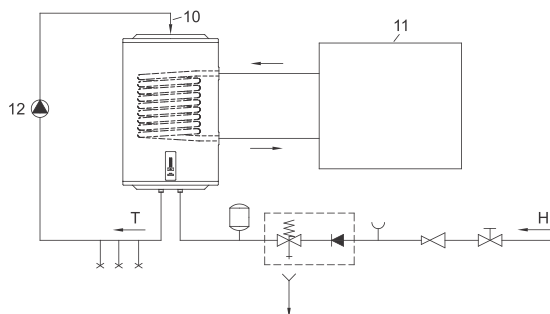
Fig. 4: Conectarea încălzitorului la sursa de energie suplimentară
