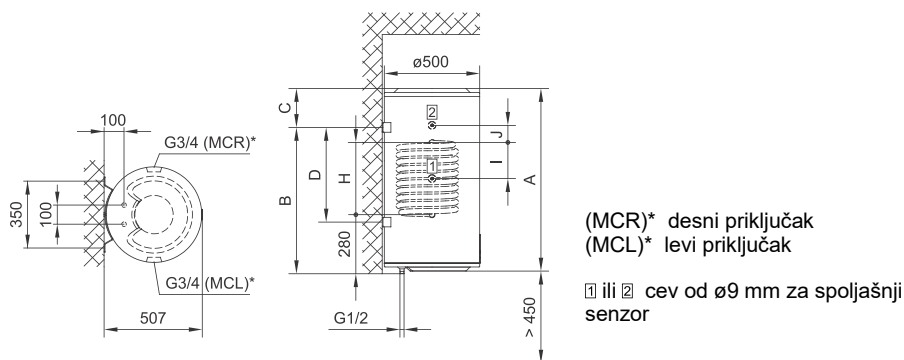
Sl. 1: Vertikalno montiranje na zid
