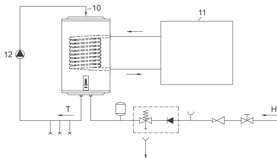
Sl. 4: Priključivanje na druge izvore grejanja
