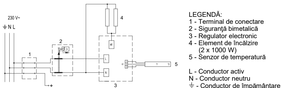
Fig. 6: Instalația electrică
