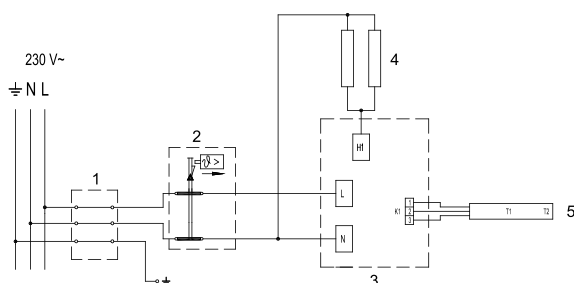
Рисунок 6: Электросхема
