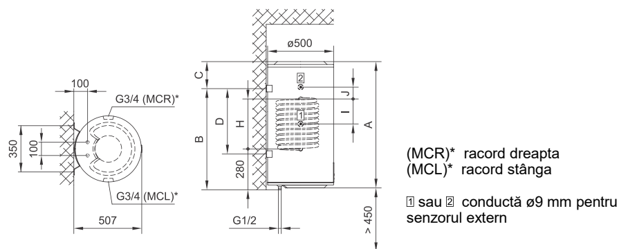
Fig. 1: Instalarea boilerului pe perete în poziție verticală
