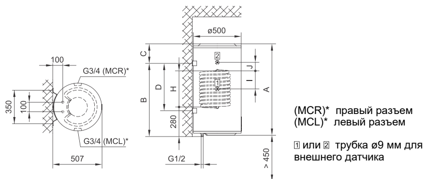
Рис. 1: Монтаж на стену в вертикальном положении
