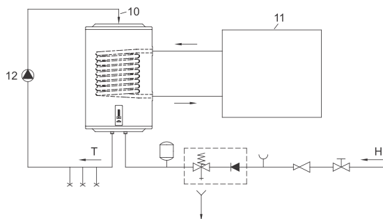
Рис. 4: Подключение водонагревателя к дополнительному источнику энергии
