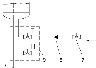
Рисунок 3: Безнапорная (открытая) система
