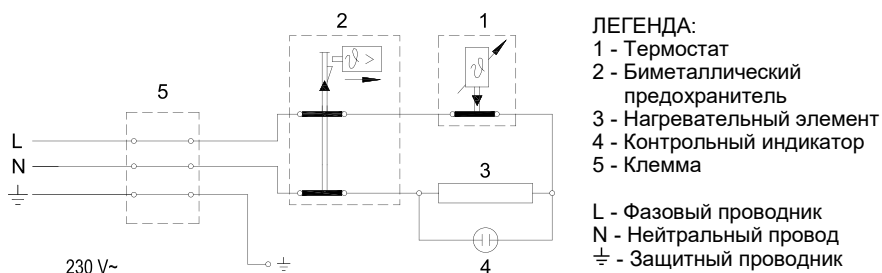
Схема электрической цепи
