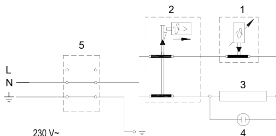
Електросхема
