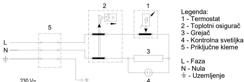
Šema povezivanja električnih provodnika
