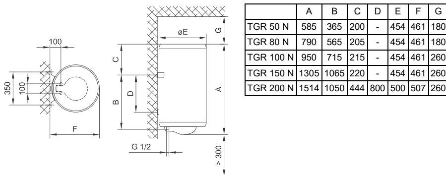
Присоединительные и монтажные размеры нагревателя [мм]
