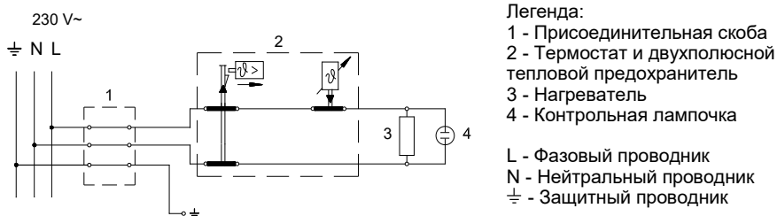
Электросхема
