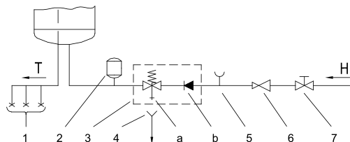
Sl. 3: Zatvoreni sistem (pod pritiskom)
