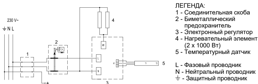
Рисунок 6: Электросхема
