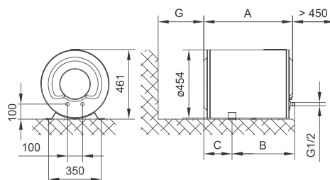
Fig. 2: Montarea orizontală pe podea
