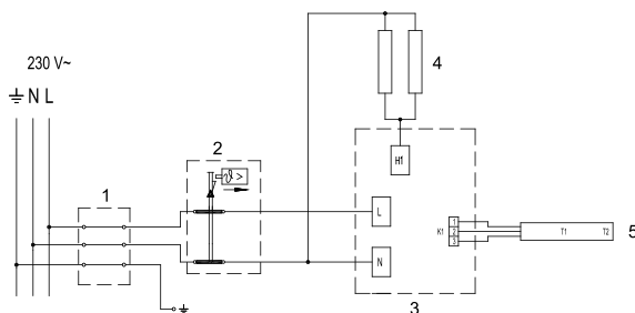
Мал. 6: Електросхема
