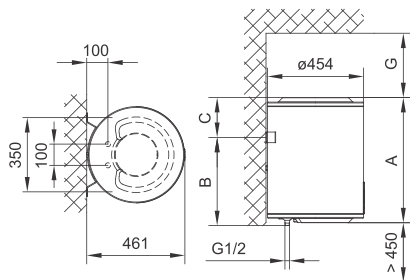
Sl. 1: Vertikalno montiranje na zid
