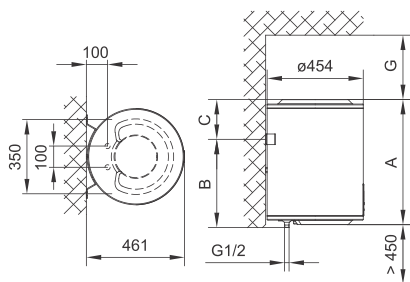
Fig. 1: Instalarea boilerului pe perete în poziție verticală
