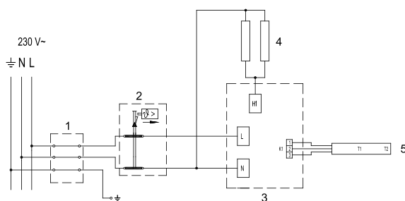
Fig. 6: Instalația electrică
