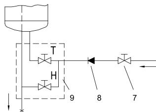
Sl. 4: Otvoreni sistem (protočni)
