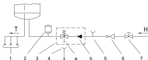
Fig. 3: Sistemul închis (presurizat)
