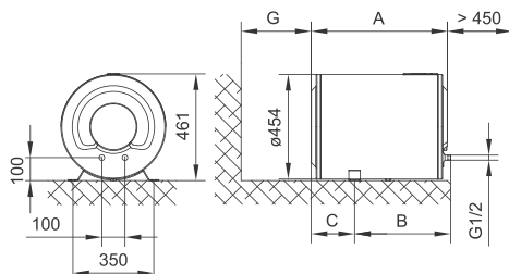
Sl. 2: Vodoravno montiranje na pod
