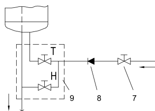
Fig. 4: Sistemul deschis (nepresurizat)
