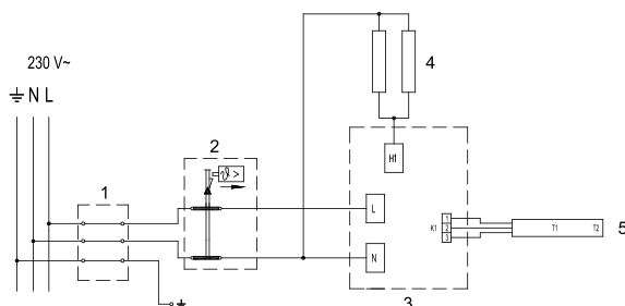
Рисунок 6: Электросхема
