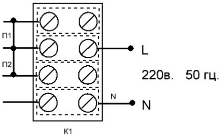
Мал.4 Схема вклучення котла в мережу 220в
