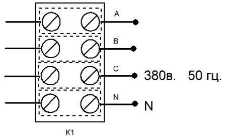
Мал.5 Схема вклучення котла в мережу 380в
