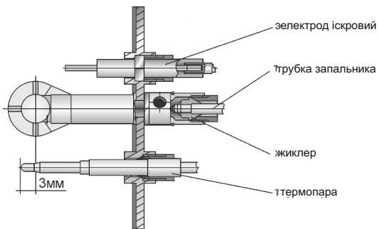
Рис. 4. Запальний пальник
