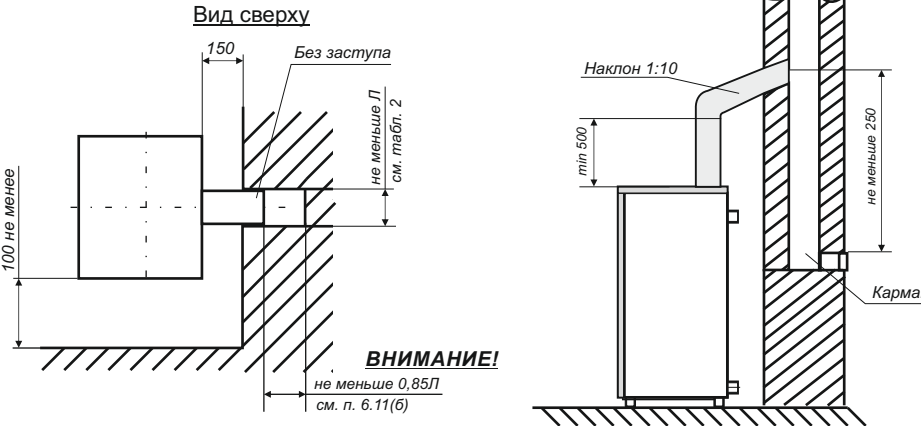
Рис. 5. Схема подключения котла к дымовому каналу и план установки котла
