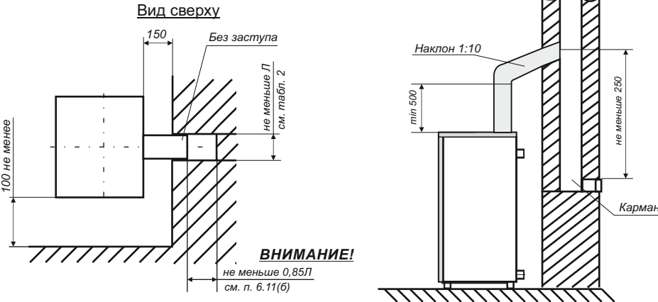
Рис. 5. Схема подключения котла к дымовому каналу и план установки котла
