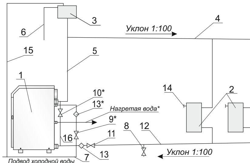
Рис. 12. Схема монтажа котла в системе отопления с природной циркуляцией теплоносителя.
