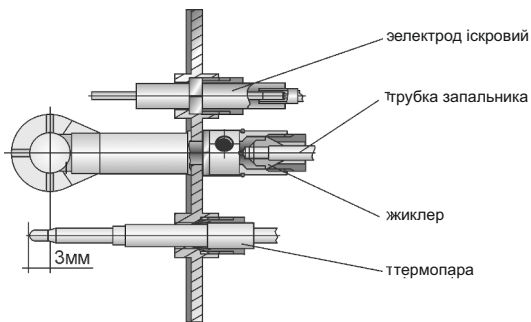
Рис. 4. Запальний палик
