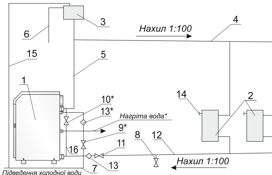
Схема монтажу котла в системі опалення з природною циркуляцією теплоносія.
