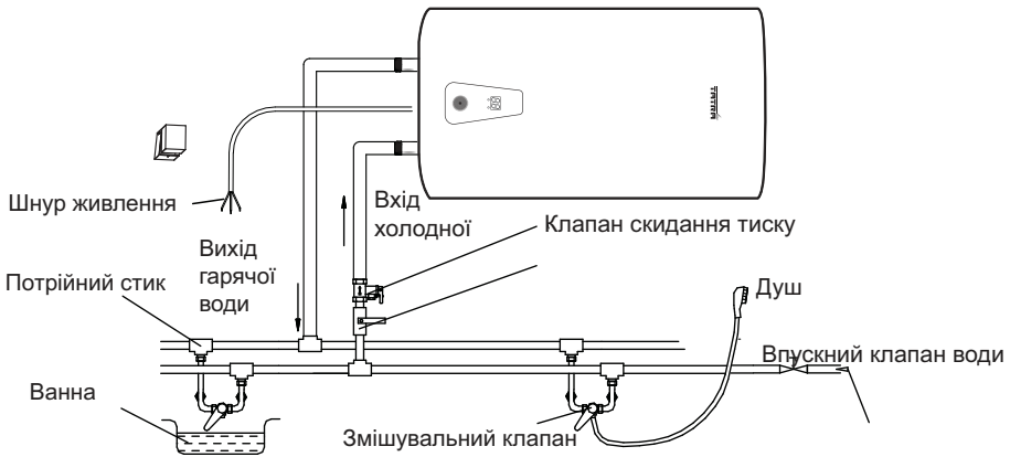
↑ ГОРИЗОНТАЛЬНИЙ МОНТАЖ
