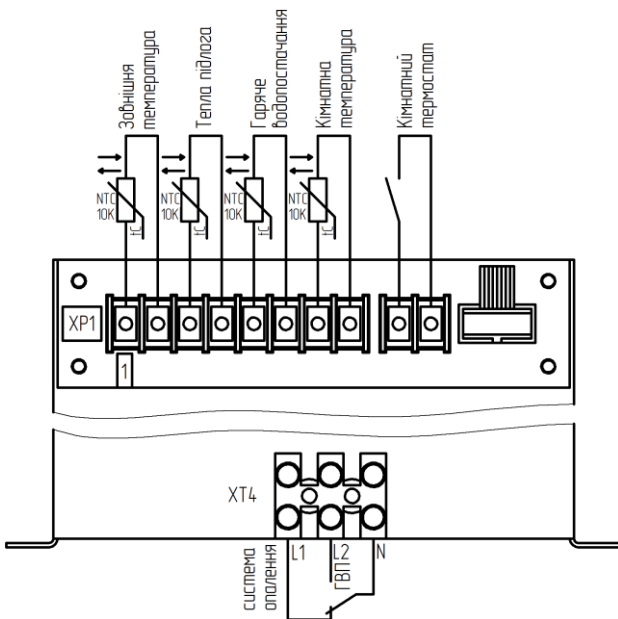
Рисунок 3 Підключення зовнішніх пристроїв
