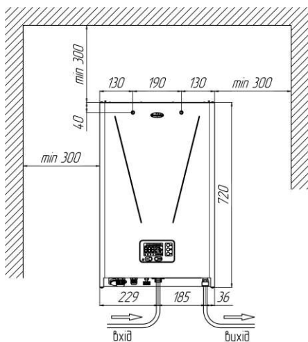
Рисунок 2. Приклад кріплення котла на стіні.
