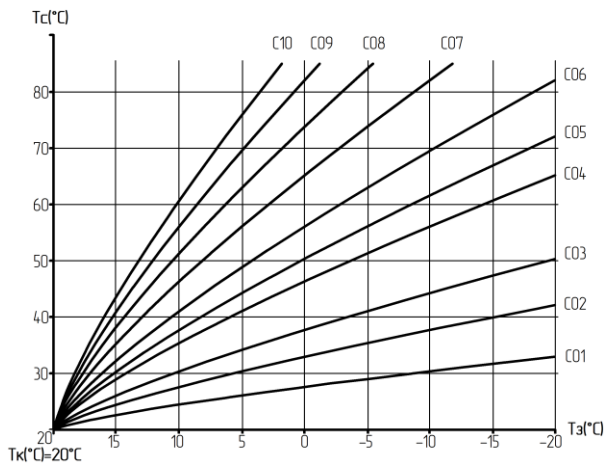
Рисунок 25 Компенсаційні криві
