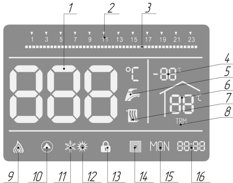
Рисунок 4. Загальний вигляд РК дисплею
