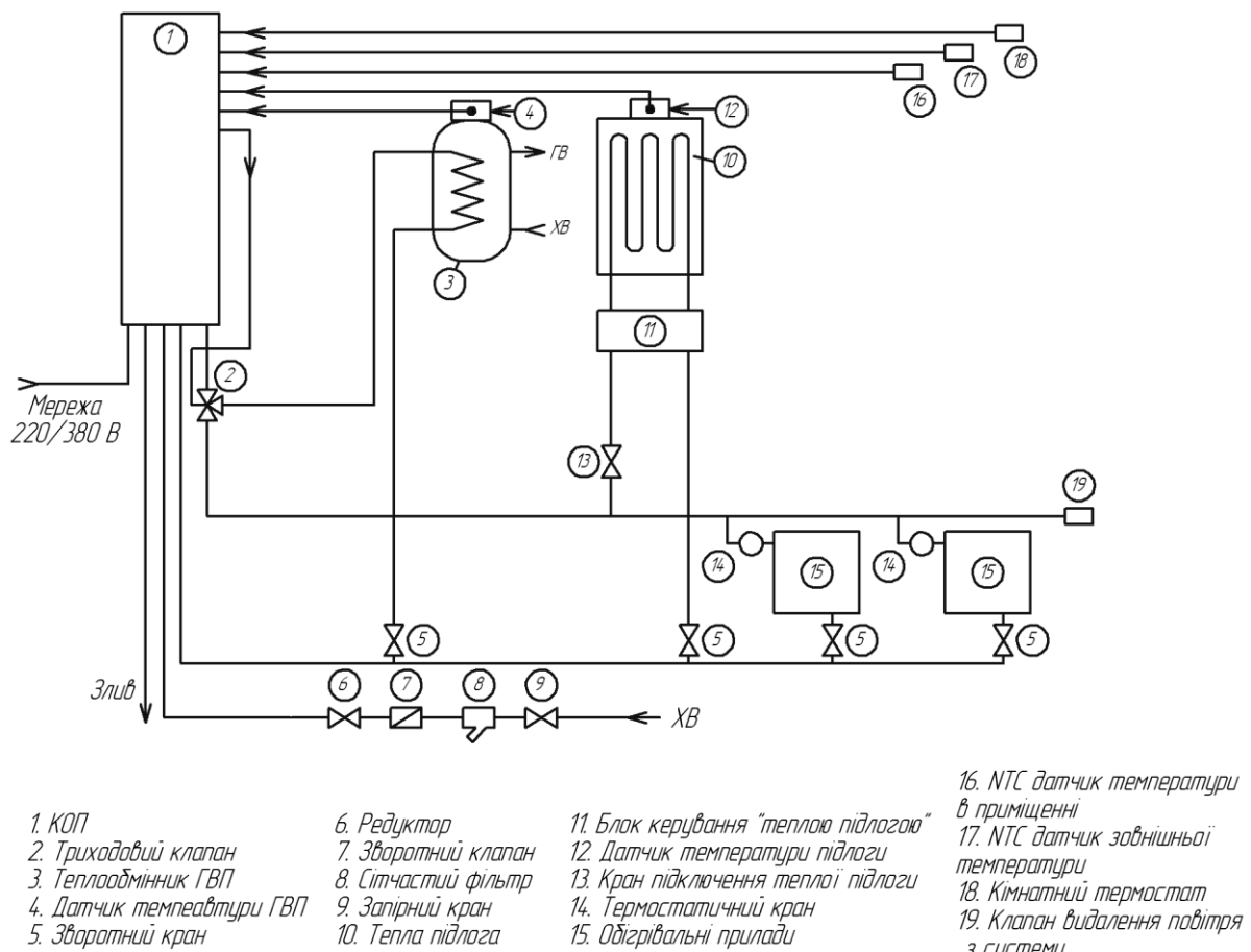
Рекомендована схема системи опалення
