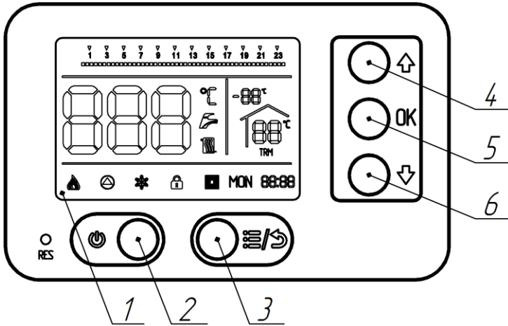
Рисунок 5 Загальний вигляд панелі керування
