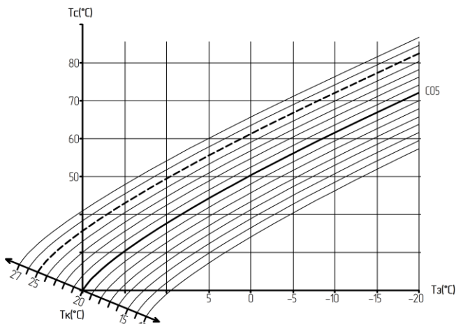
Рисунок 26 Приклад зміщення компенсаційної кривої
